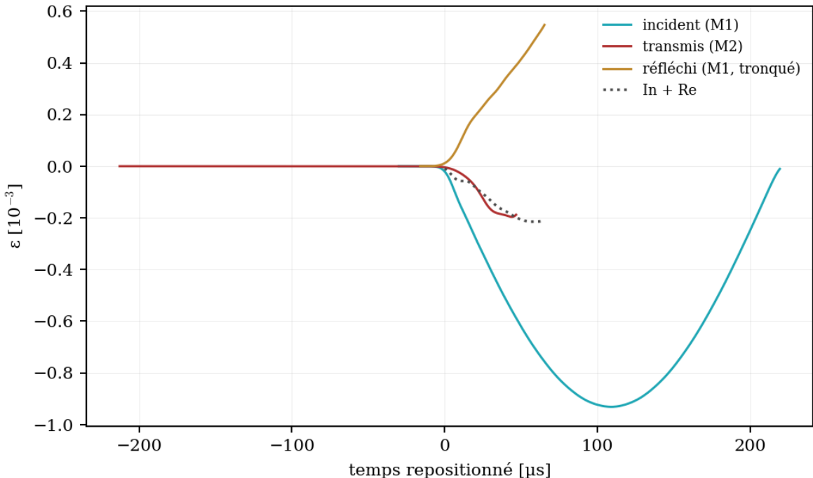
(b) équilibre dynamique In+Re vs Tr (fig. 24)
