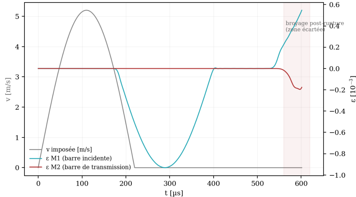
(a) SHPB adaptatif — impulsion et jauges (fig. 23)
