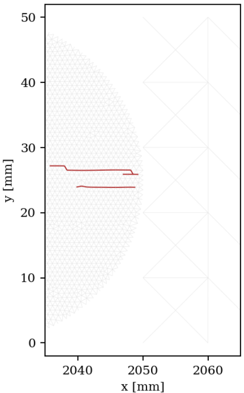
(c) disque à t \approx 470 μs — rupture franche
