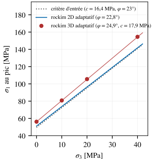
(a) enveloppe de Coulomb
