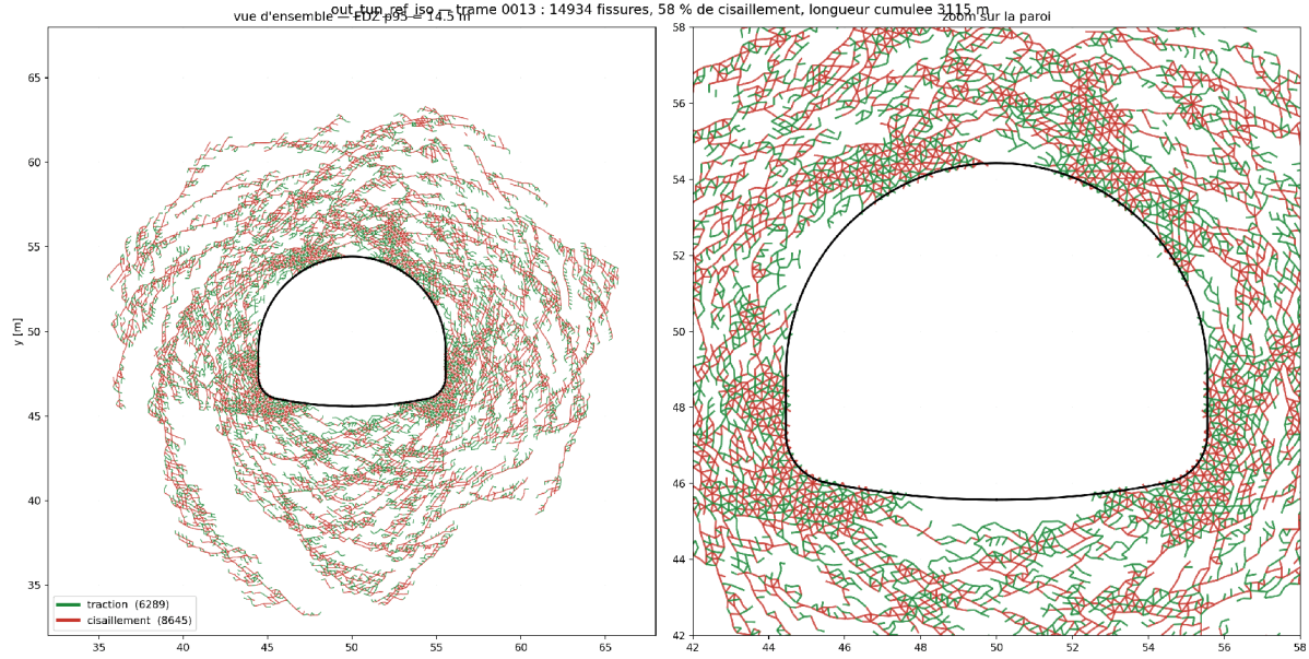
FIGURE 35 – Réseau de fissures du cas de référence, traction en vert et cisaillement en rouge : vue d'ensemble et zoom sur la paroi. L'anneau est La figure classe en deux modes, selon la part dominante (traction en vert, 6 289 ; cisaillement en rouge, 8 645), et non en trois comme le texte. Anneau quasi circulaireet , granulé à l'échelle de l'élément près de la paroi.
