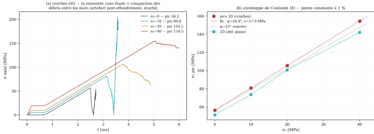
FIGURE 22 – Triaxial 3D adaptatif. (a) Contrainte axiale ; la remontée finale à 10 MPa est une compaction de débris. (b) Enveloppe linéaire, \varphi = 24,9^\circ , c = 17,9 MPa, pour 23^\circ et 16,4 MPa en entrée.
