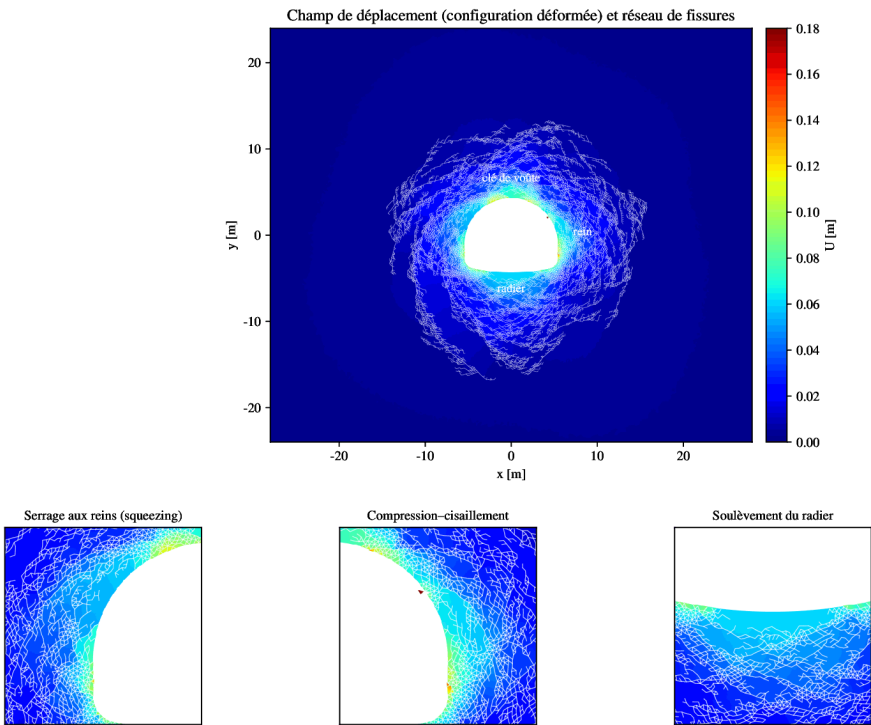
Tunnel de Hutou Beishan — leur fig. 11 ( \sigma = 5 \text{ MPa} , \lambda = 1 ) : U paroi 0.148 m, débris 0.389 m (publié : 0,347)
