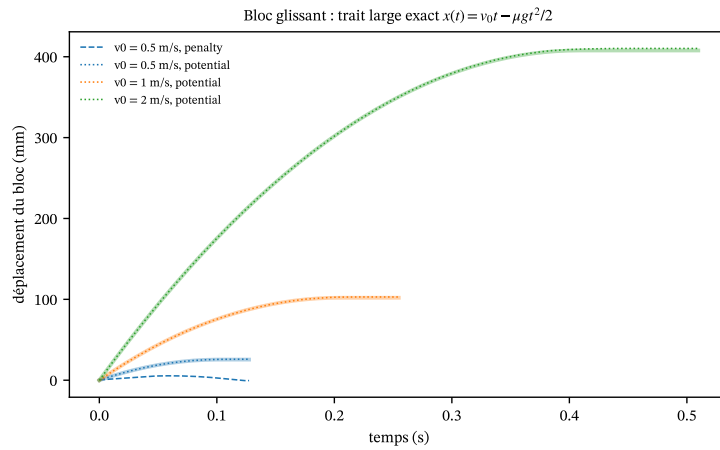
FIGURE 13 – Bloc glissant : déplacement contre en fonction du temps pour trois vitesses initiales, contact par potentiel et par pénalité nœud-face, solution exacte en trait large.
