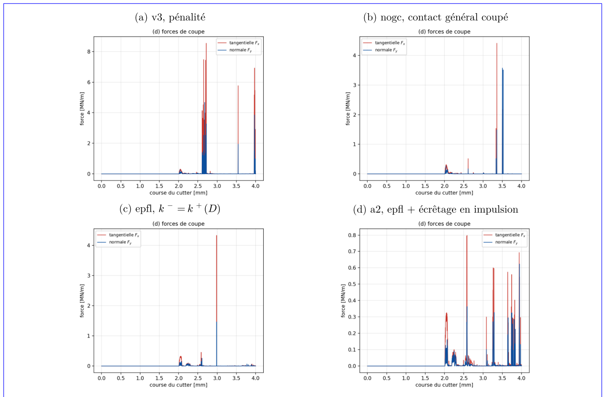
FIGURE 45 – Forces de coupe tangentielle (rouge) et normale (bleu) en fonction de la course, calculs d'août 2026, planches d'archive recadrées : (a) v3; (b) contact général coupé; (c) pénalité de compression de Ghesquière-Diérckx et al.; (d) même pénalité et écrêtage en impulsion.
