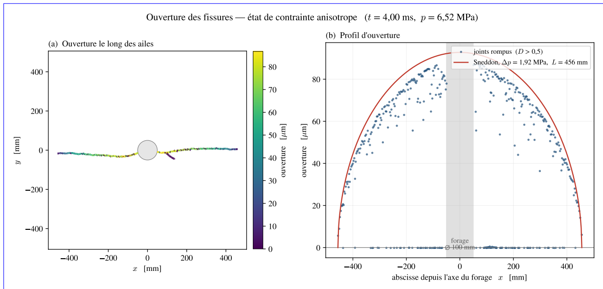
FIGURE 28 – Ouverture des fissures à t = 4 ms, état anisotrope, reconstruite lèvre à lèvre, et ellipse de Sneddon ( \Delta p = 1,92 MPa, L = 456 mm) : 89,0 \mu m mesurés pour 92,8 \mu m prédits. Les points à ouverture nulle sont des joints refermés.
