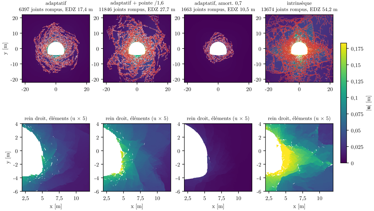
FIGURE 43 – Rejeu sur maillage réduit (binaire f0209ef0209ef), quatre variantes à 0,23 s après le début du relâchement. En haut, norme du déplacement sur la configuration déformée et joints rompus (rouge : cisaillement ; blanc : traction). En bas, rein droit en rendu éléments, déplacements amplifiés 5 fois.
