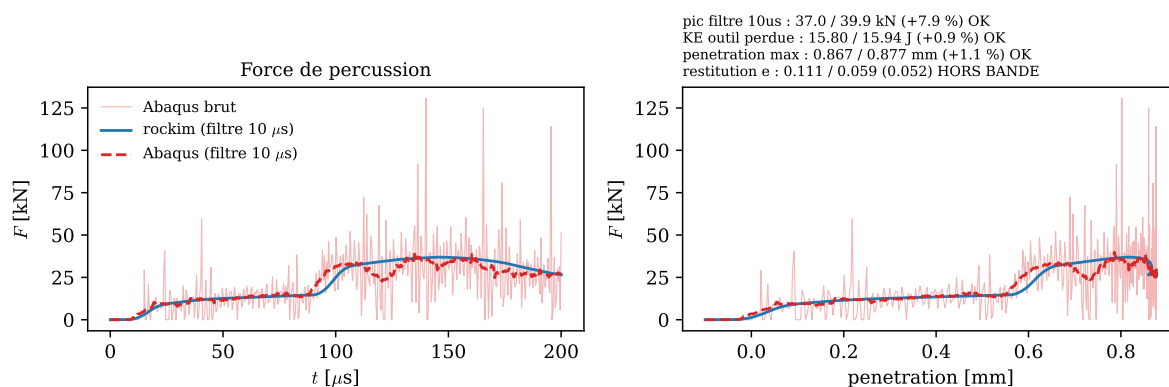
FIGURE 61 – Validation croisée Comparaison de code à code entre rockim et Abaqus/Explicit, loi de Saksala 2011, même maillage : force de percussion filtrée contre le en fonction du temps et de la pénétration.
