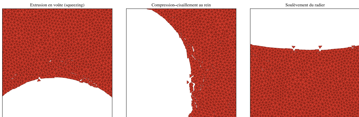
FIGURE 40 – Modes de ruine en rendu éléments, k_{\text{tip}} = 1,6 , t = 0,7 s (les vides sont en blanc) : extrusion en voûte, compression-cisaillement au rein, soulèvement du radier, les trois modes décrits par Wang et al.
