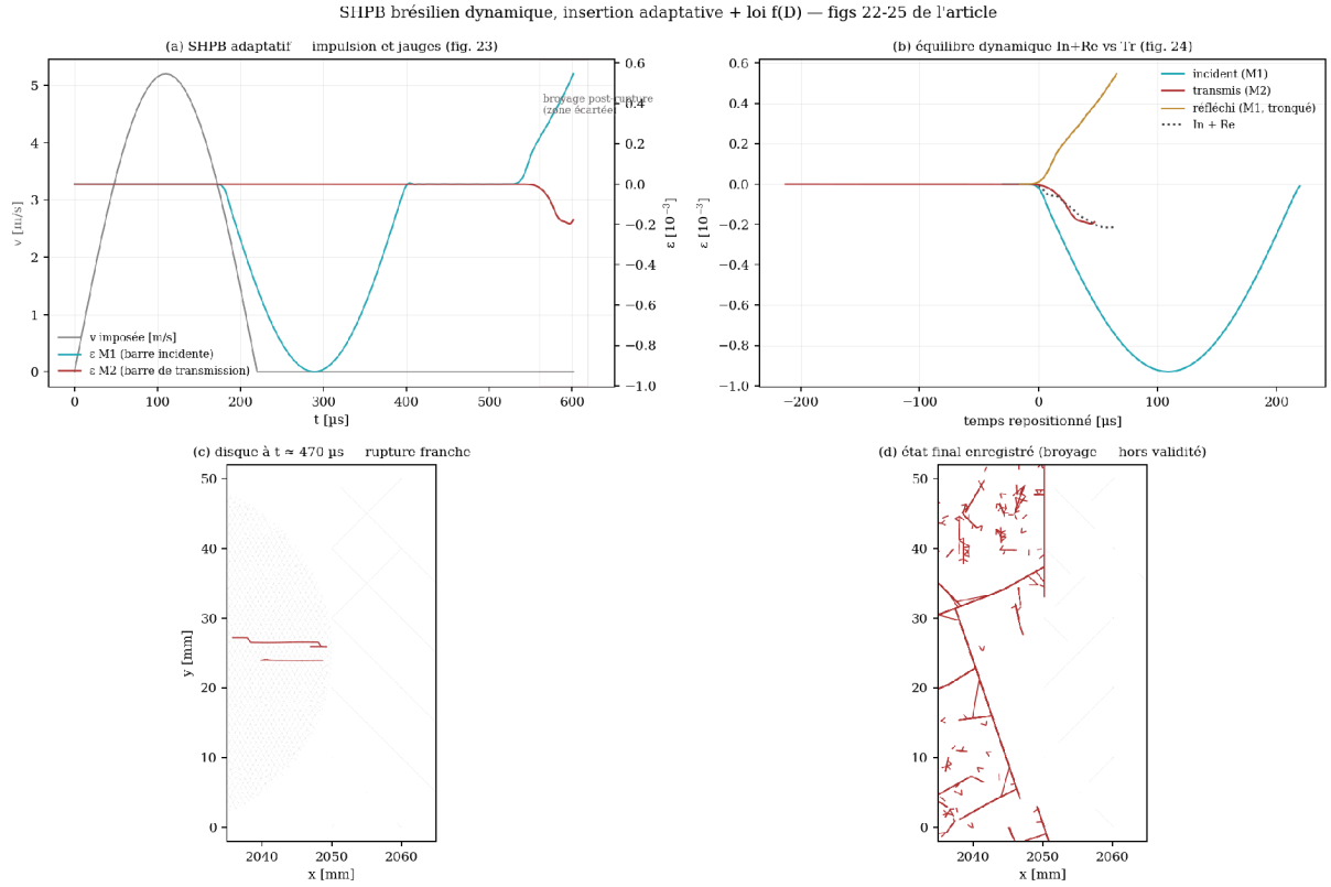
FIGURE 24 – Brésilien dynamique adaptatif. (a) Vitesse imposée et déformations aux jauges. (b) Équilibre \varepsilon_I + \varepsilon_R \approx \varepsilon_T avant rupture. (c) Fente centrale à 470 \mu s. (d) Broyage tardif, hors validité.
