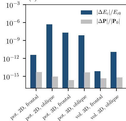
(c) écarts relatifs en fin d'essai
