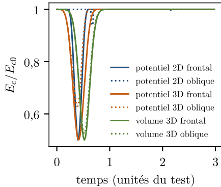
(b) énergie cinétique
