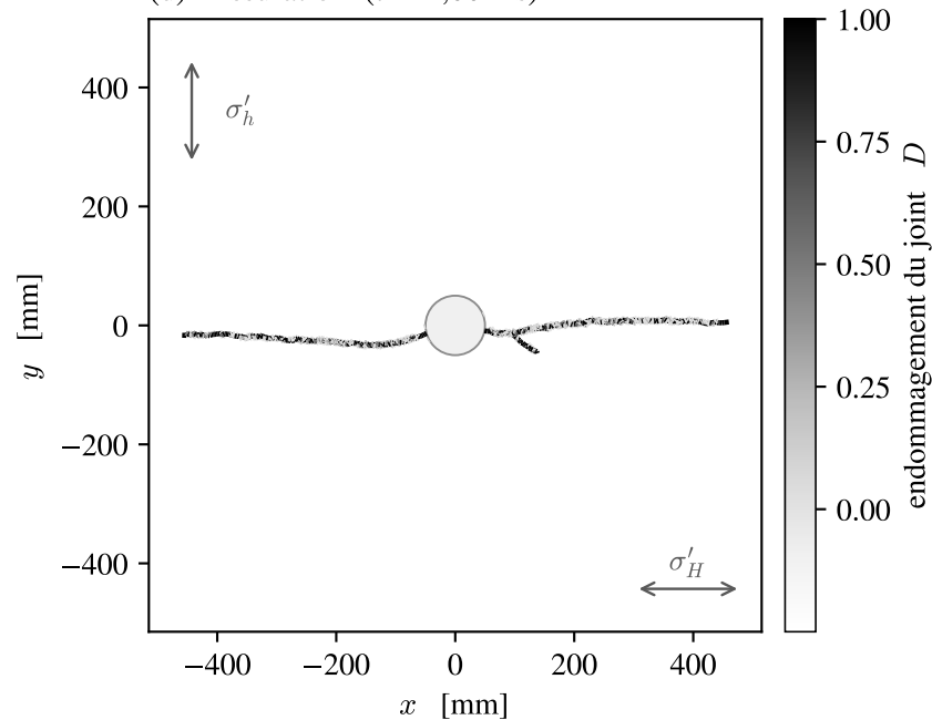
(d) Fissuration ( t = 4,00 ms)
