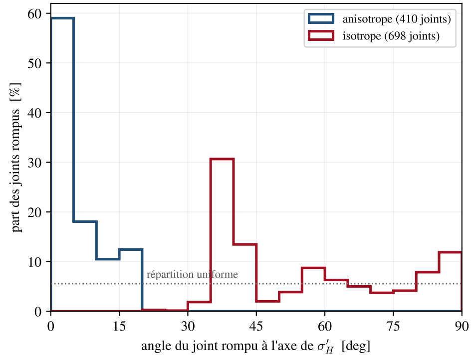
(b) Distribution angulaire de la fissuration
