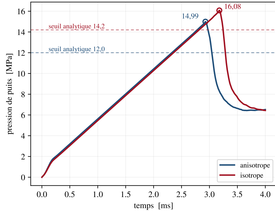
(a) Pression de puits
