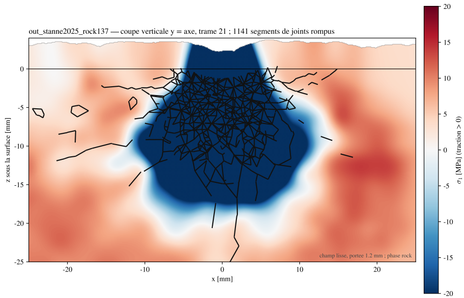
FIGURE 52 – Contrainte principale majeure (traction positive) en coupe verticale par l'axe à 300 \mu s, avec les traces des joints rompus : noyau comprimé sous l'insert, couronne en traction.
