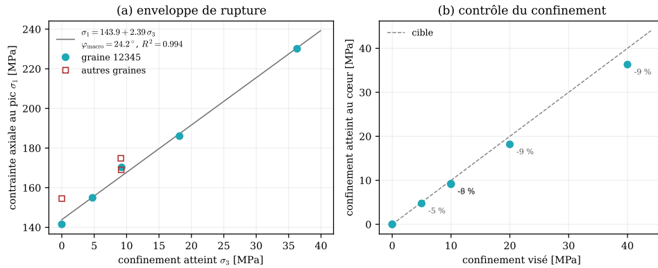
FIGURE 61 – Enveloppe du jeu de juillet. (a) Ajustement de Mohr-Coulomb des pics, angle macroscopique 24,2^\circ . (b) Confinement atteint contre visé, sous-tiré de 5 à 9 %.
