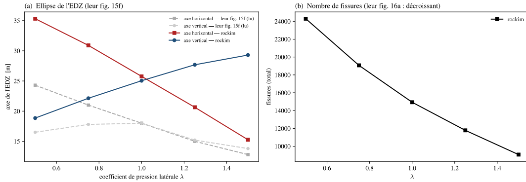
FIGURE 37 – Balayage du rapport de contraintes \lambda : (a) axes de l'EDZ ( 2a_h , 2a_v ) et valeurs lues sur la figure 15f de Wang et al. ; (b) nombre de fissures, qui décroît d'un facteur 2,7 dans les deux codes.
