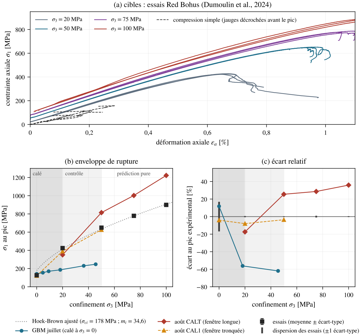
FIGURE 62 – Calibration Red Bohus. (a) Essais de Dumoulin et al. (b) Enveloppe : le jeu de juillet sous-estime le confinement, celui d’août le surestime au-delà de 50 MPa. (c) Écart au pic expérimental.
