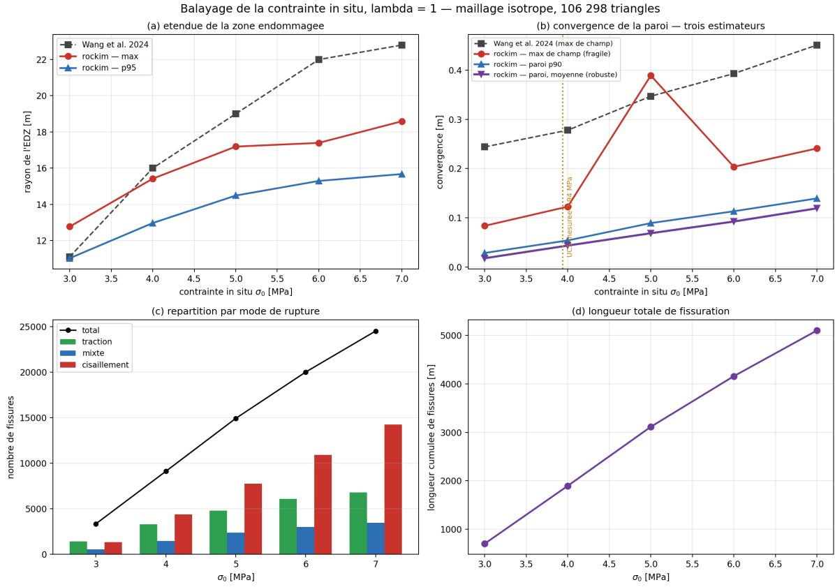
FIGURE 36 – Balayage de la contrainte in situ ( \lambda = 1 ) : rayon d'EDZ comparé aux valeurs lues chez Wang et al., convergence de paroi selon trois estimateurs, répartition des modes et longueur fissurée.
