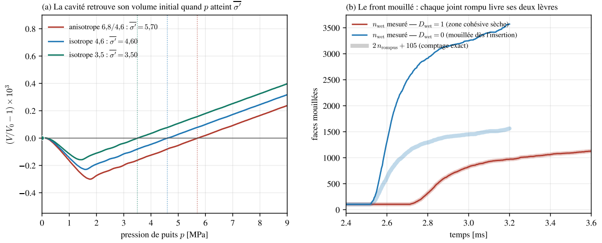
FIGURE 27 – Contrôles du couplage. (a) Variation relative du volume de la cavité en fonction de la pression : la cavité se referme puis retrouve son volume initial quand la pression égale la contrainte moyenne in situ. (b) Le front mouillé compte exactement deux lèvres par joint rompu à D_{\text{wet}} = 1 ; à D_{\text{wet}} = 0 , il suit les insertions.
