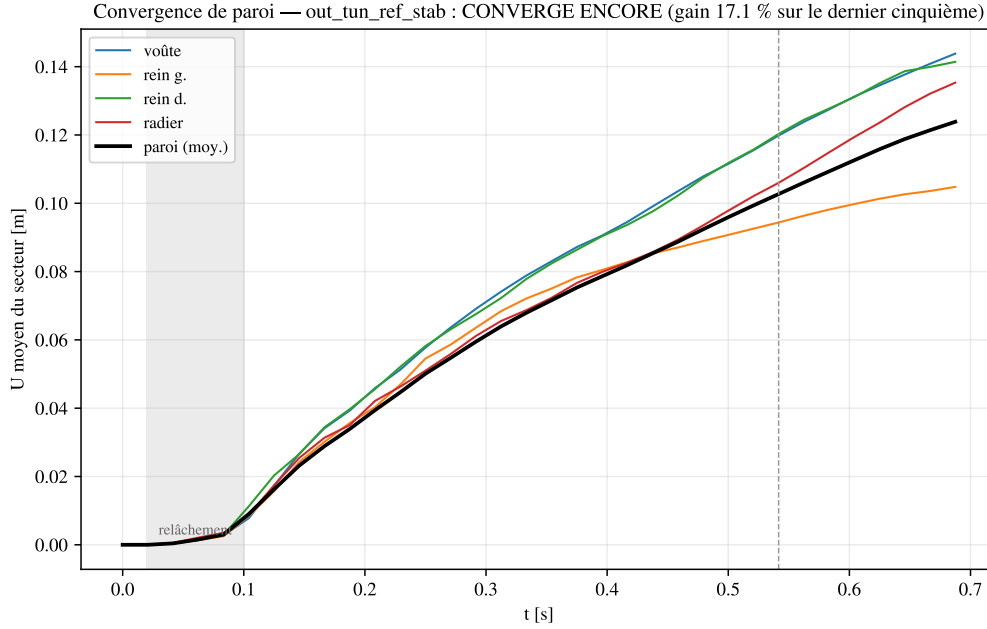
FIGURE 42 – Convergence de paroi par secteur, calcul de référence prolongé : la paroi converge encore à 0,69 s (17 % du déplacement sur le dernier cinquième), d'où la comparaison à temps égal.
