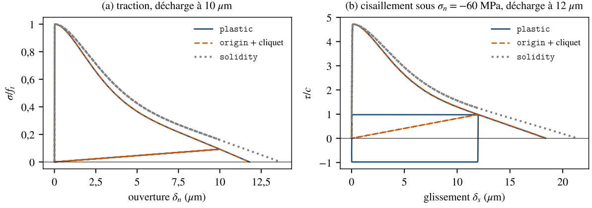
FIGURE 3 – Joint isolé, trois branches de décharge, rejoué. (a) Traction avec décharge à 10 \mu\text{m} . (b) Cisaillement sous \sigma_n = -60 \text{ MPa} avec décharge à 12 \mu\text{m} : seule la branche plastic conserve un glissement résiduel.
