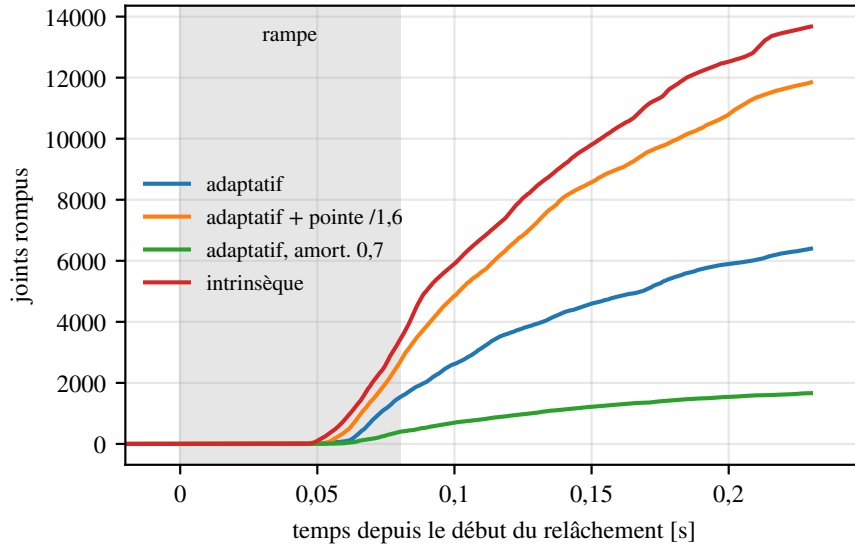
FIGURE 45 – Nombre de joints rompus en fonction du temps depuis le début du relâchement (rejeu du 6 octobre 2026). La fissuration démarre aux deux tiers de la rampe et ne sature dans aucune variante à 0,23 s.
