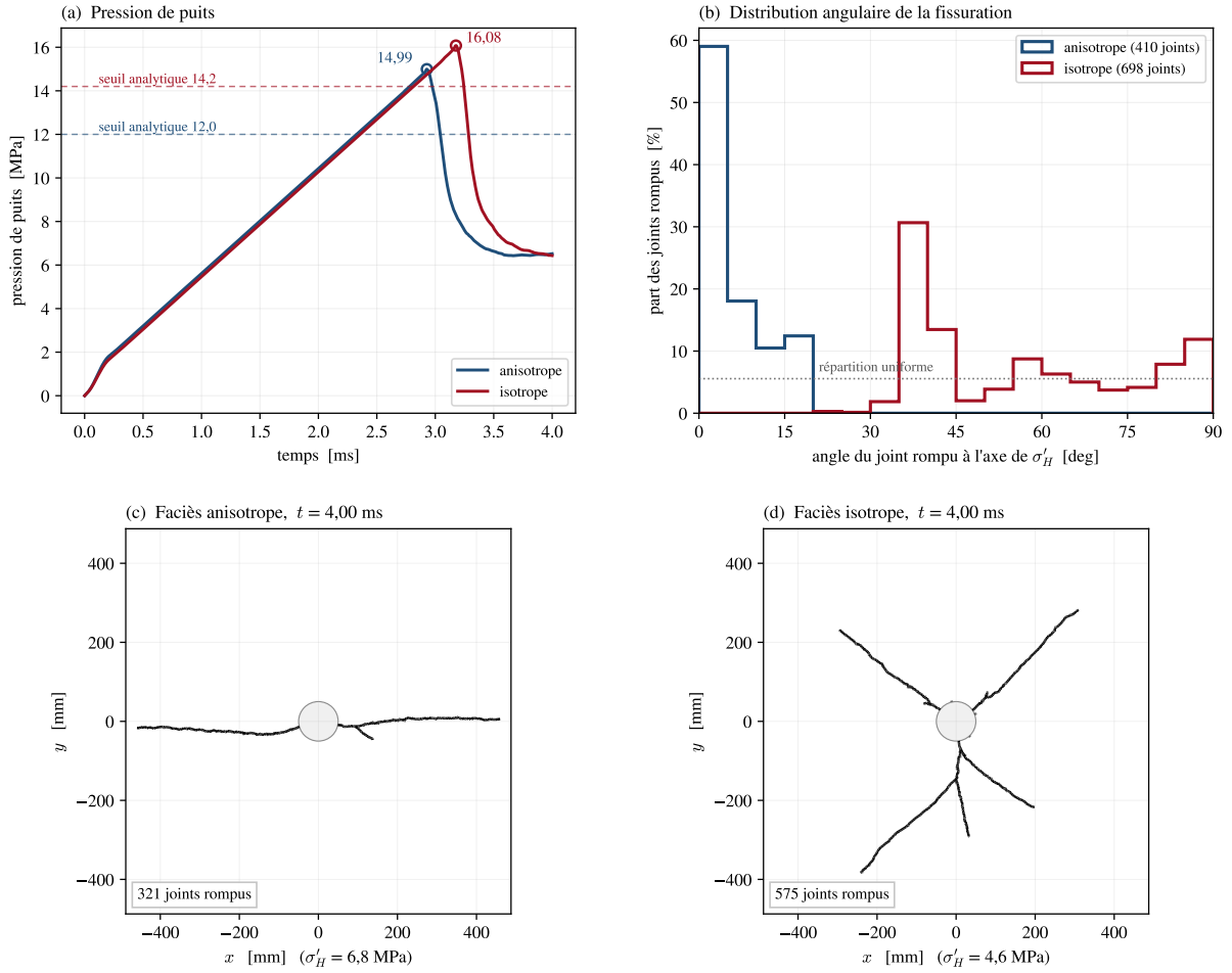
FIGURE 31 – Effet de l'état de contrainte lointain, mêmes maillage, roche et pompe : (a) pression de puits contre les seuils analytiques de 12,0 et 14,2 MPa ; (b) distribution angulaire des joints rompus ; (c, d) faciès en deux ailes (anisotrope, 321 joints rompus) et en étoile radiale (isotrope, 575 joints rompus) à 4 ms.
