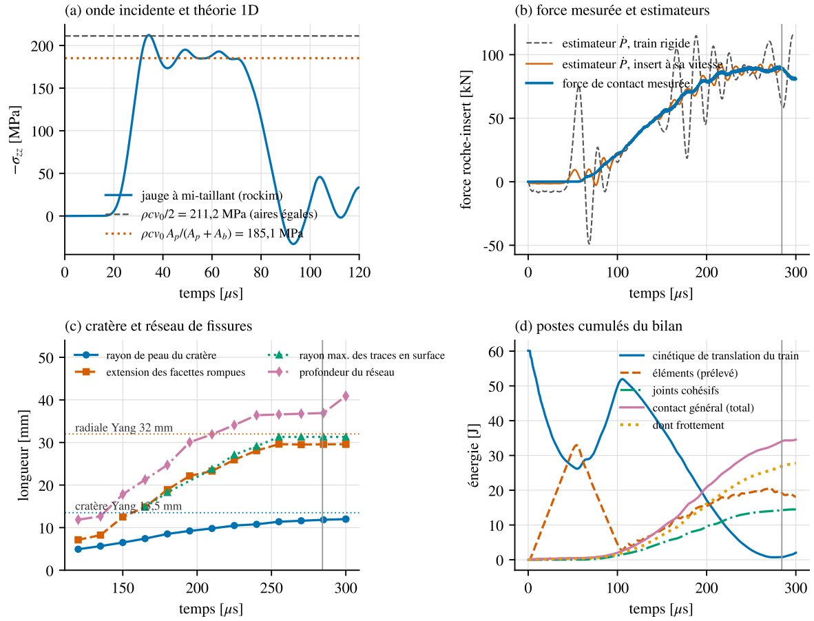
FIGURE 47 – Réplique St Anne : (a) onde à la jauge et théorie unidimensionnelle ; (b) force insert-roche mesurée et estimateurs ; (c) croissance du cratère et du réseau ; (d) postes du bilan d'énergie. Trait vertical : fin de charge.
