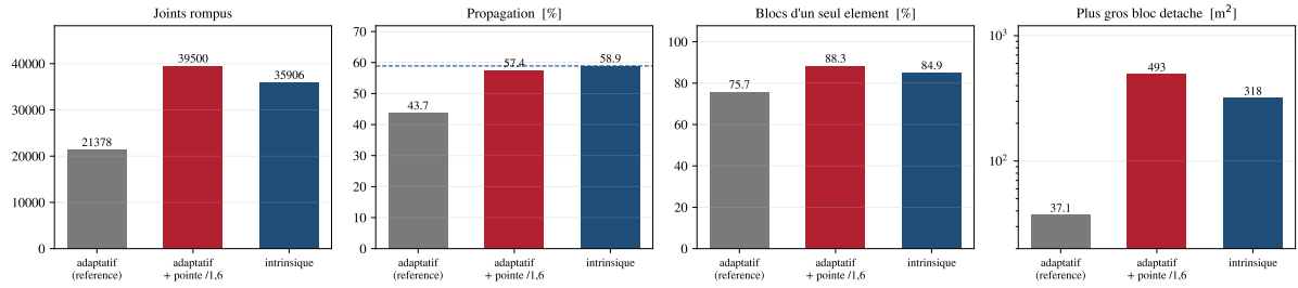
FIGURE 40 – Trois schémas d'insertion à temps égal depuis le relâchement : joints rompus, part de propagation, part de blocs d'un seul élément et plus gros bloc. Le facteur de pointe amène l'adaptative à la part de propagation de l'intrinsèque (57,4 % contre 58,9 %).
