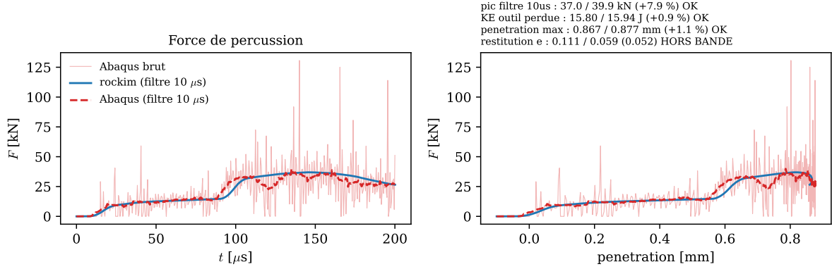
FIGURE 59 – Validation croisée rockim et Abaqus/Explicit, loi de Saksala 2011, même maillage : force de percussion filtrée contre le temps et la pénétration.
