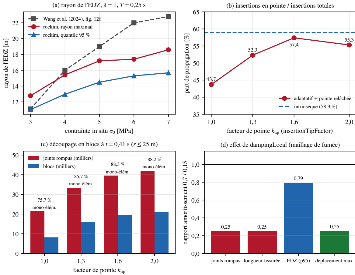
FIGURE 43 – Synthèse du banc du tunnel : (a) rayon d'EDZ en fonction de \sigma_0 , rockim et Wang et al. ; (b) part de propagation en fonction de k_{tip} ; (c) joints rompus et blocs à 0,41 s en fonction de k_{tip} ; (d) rapports entre amortissements 0,7 et 0,15.
