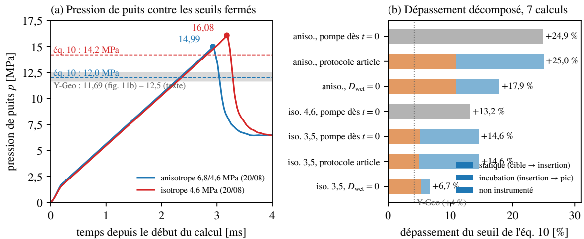
FIGURE 29 – (a) Pression de puits des deux calculs de référence (maille de 3 mm), contre la formule de Hubbert et Willis (tirets) et la valeur de Y-Geo (bande grise) ; traits fins : rejoux du 6 octobre 2026 sur maillages grossiers. (b) Dépassement du seuil des sept calculs, décomposé en part statique et part d'incubation.
