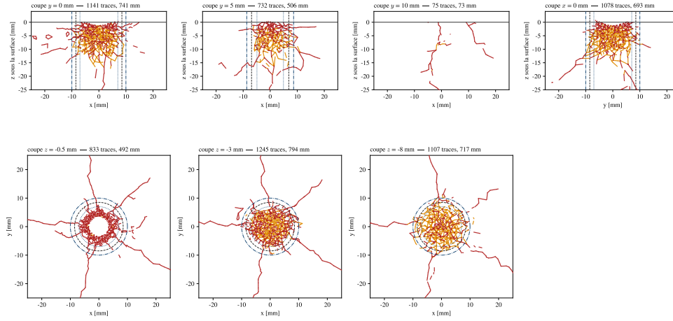
FIGURE 50 – Réplique St Anne à 300 \mu s : traces exactes des facettes rompues dans sept plans de coupe ; rouge traction, orange cisaillement.
