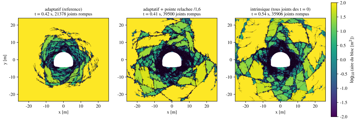
FIGURE 39 – Taille des blocs intacts (aire en échelle logarithmique) pour l'insertion adaptative, l'adaptative avec k_{\text{tip}} = 1,6 et l'intrinsèque : l'adaptative granule un anneau, les deux autres découpent des blocs polygonaux de dizaines à centaines de m 2 .
