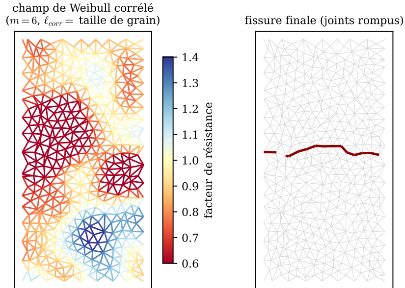
FIGURE 64 – Champ de Weibull corrélé sur les joints ( m = 6 , longueur de corrélation égale à la taille de grain) et fissure de traction finale, qui suit la bande la plus faible.
