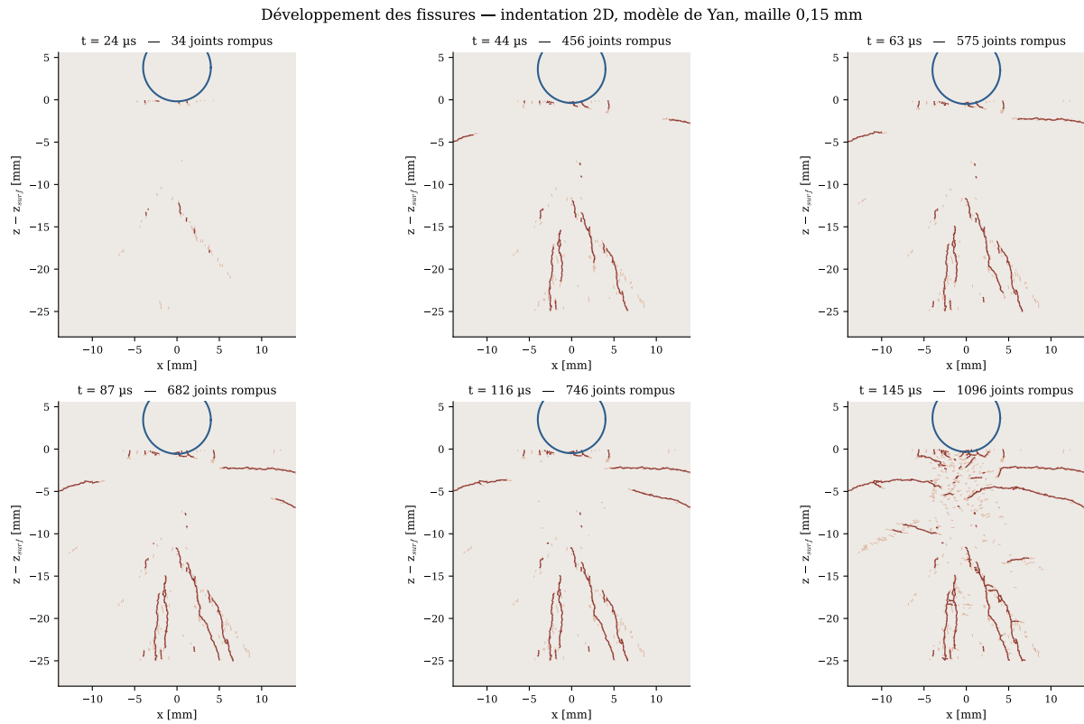
FIGURE 58 – Indentation 2D d’un bouton sphérique, modèle de Yan, maille de 0,15 mm : fissures médianes, puis latérales, puis broyage sous le bouton à la décharge.
