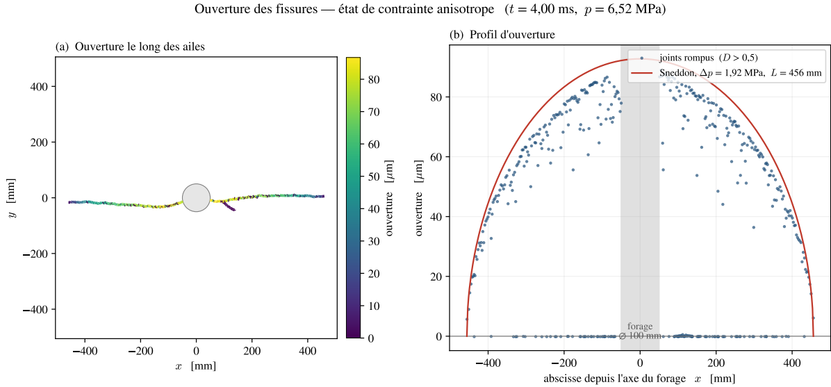
FIGURE 28 – Ouverture des fissures à t = 4 ms ( p = 6,52 MPa), état anisotrope, reconstruite lèvre à lèvre, contre l'ellipse de Sneddon ( \Delta p = p - \sigma'_h = 1,92 MPa, L = 456 mm) : 89,0 \mu\text{m} mesurés pour 92,7 \mu\text{m} prédits. Les points à ouverture nulle sont des joints refermés.
