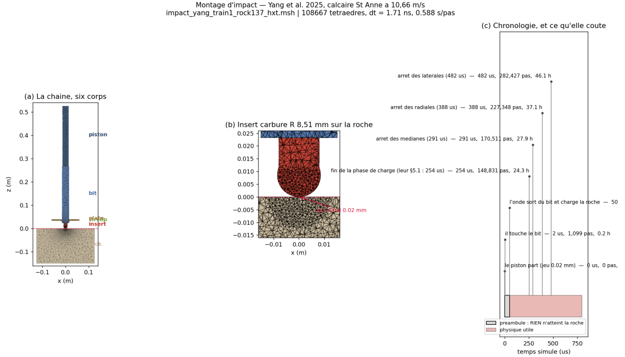
FIGURE 46 – Montage de la réplique St Anne : chaîne de six corps, insert en carbure posé à 0,02 mm de la roche, et coût en temps de calcul des événements de la chronologie.
