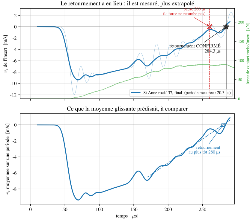
FIGURE 54 – Datation de la fin de charge : la vitesse de l’insert s’annule à 260 \mu\text{s} sans décharge, puis s’inverse à 284,3 \mu\text{s} .
