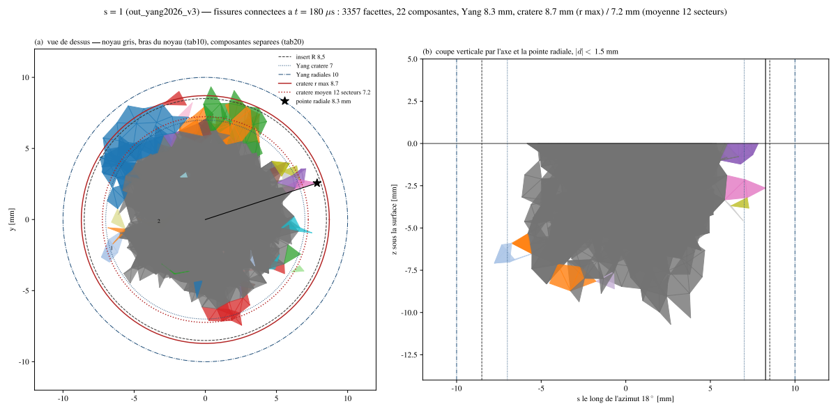
FIGURE 55 – Réplique Kuru, maillage fin, à 180 \mu s : réseau connecté vu de dessus et en coupe ; noyau dense de 7 à 9 mm, pas d'étoile radiale.
