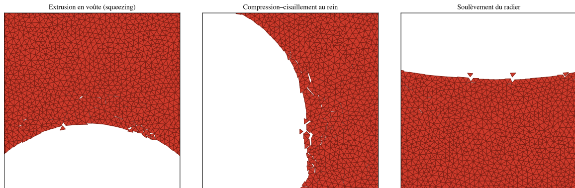
FIGURE 41 – Modes de ruine en rendu éléments, k_{tip} = 1,6 , t = 0,7 s (les vides sont en blanc) : extrusion en voûte, compression-cisaillement au rein, soulèvement du radier, les trois modes décrits par Wang et al.
