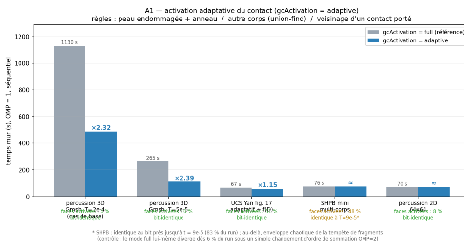
FIGURE 65 – Temps de calcul avec et sans activation adaptative du contact sur cinq cas, à un fil, avec la part de faces activées.
