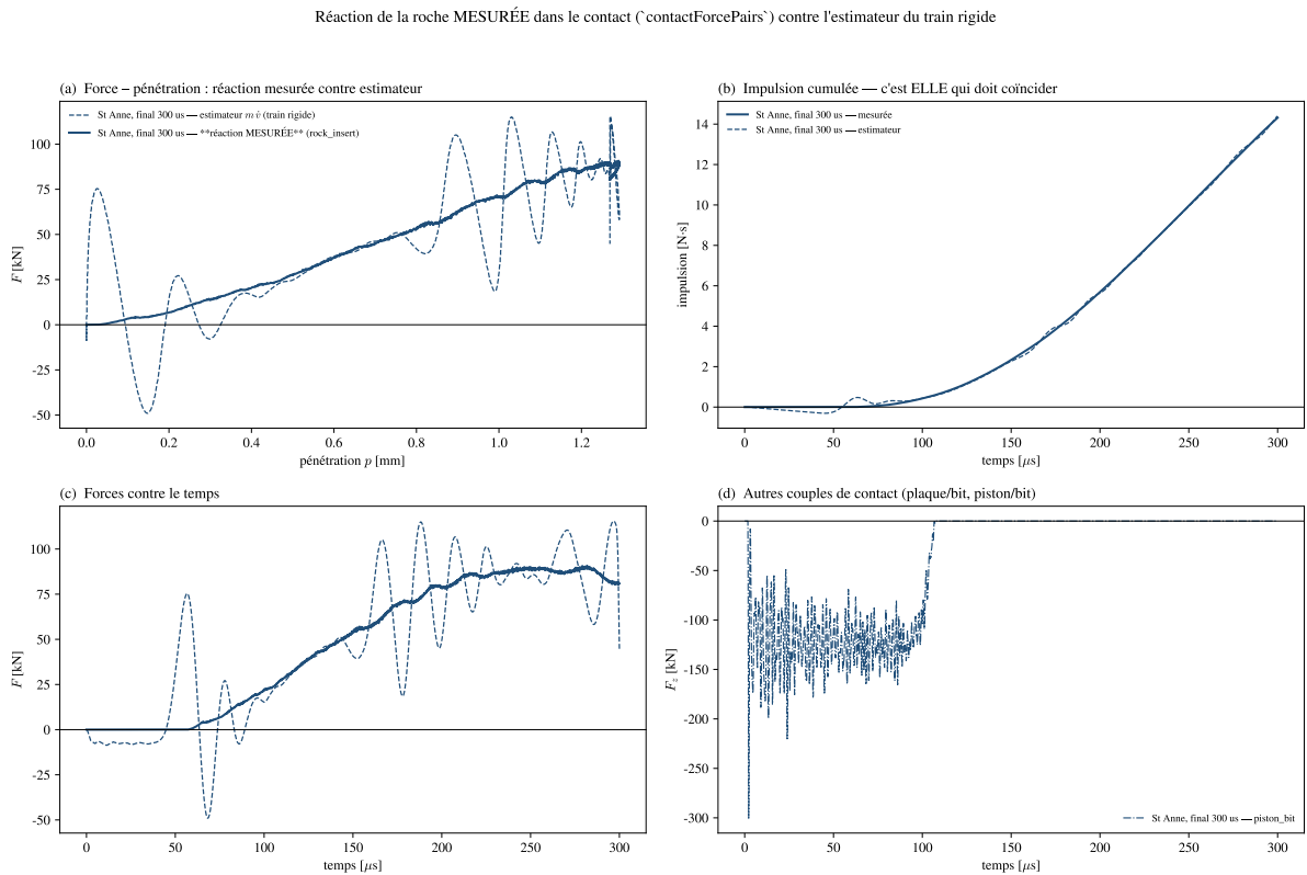
FIGURE 53 – Réplique St Anne : force de contact insert-roche mesurée contre l'estimateur du train rigide, en fonction de la pénétration et du temps, impulsions cumulées et autres paires de contact.
