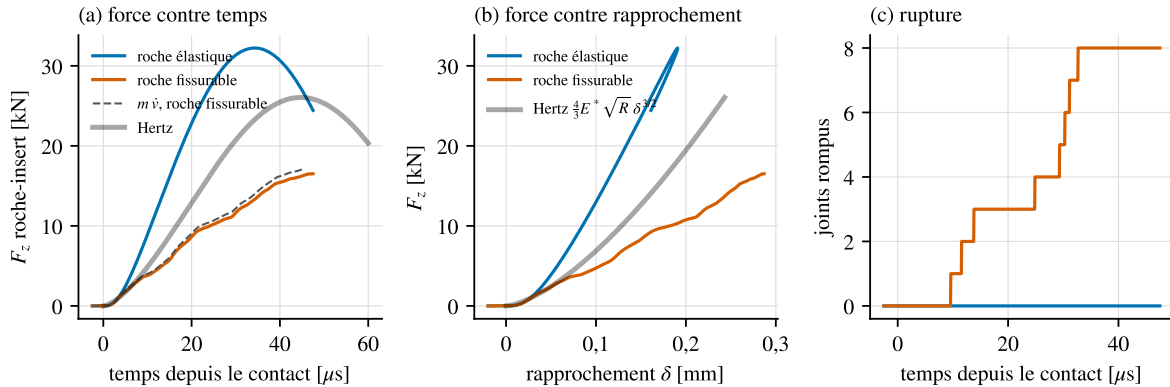
FIGURE 57 – Impact d'un insert en carbure sur roche élastique et fissurable, 50 \mu\text{s} , rejoué : force de contact contre Hertz ; le contact maillé est trop raide, l'adoucissement des joints l'assouplit avant toute rupture.
