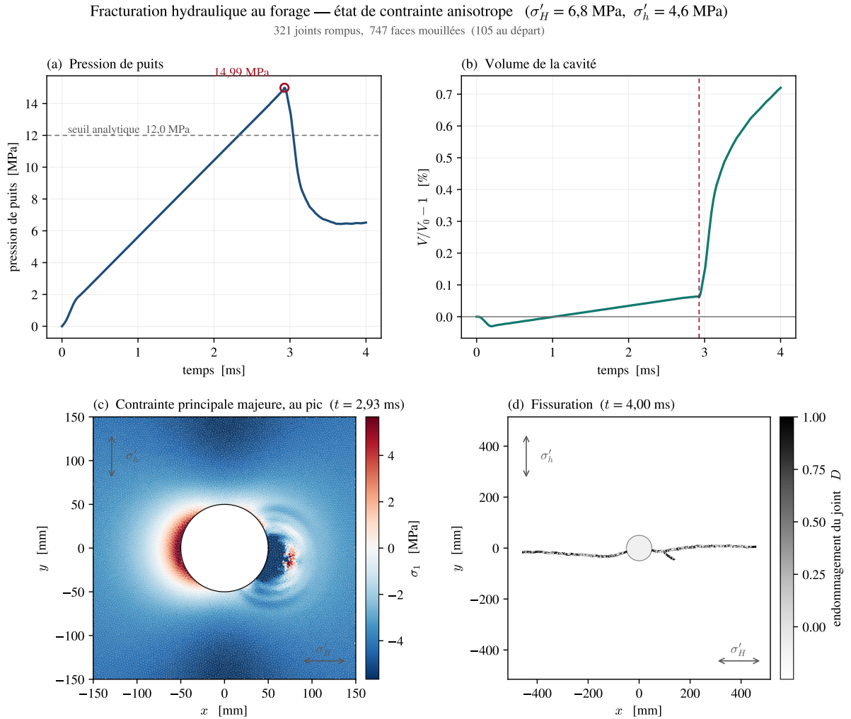
FIGURE 30 – Forage sous injection, état anisotrope ( \sigma'_H = 6,8 , \sigma'_h = 4,6 MPa) : (a) pression de puits, pic de 14,99 MPa contre 12,0 MPa pour la formule de Hubbert et Willis ; (b) volume de la cavité ; (c) contrainte principale majeure au pic ; (d) fissuration à 4 ms, deux ailes de 456 mm sur l'axe de \sigma'_H .
