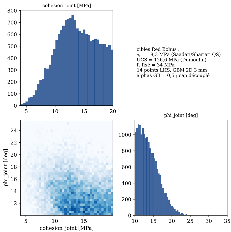
FIGURE 60 – Postérieur de la calibration de juillet, modèle à grains 2D : angle de frottement des joints médian 13,4^\circ , tronqué par la borne a priori ; cohésion peu contrainte.
