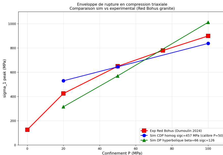
FIGURE 63 – Abaqus, lois continues : le modèle d'endommagement plastique calé à 50 MPa donne une enveloppe linéaire, le Drucker-Prager hyperbolique une courbure de sens contraire.
