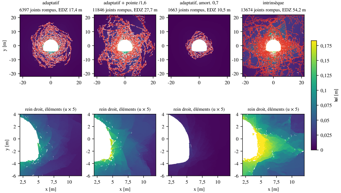
FIGURE 44 – Rejeu sur maillage réduit (binaire f0209ef), quatre variantes à 0,23 s après le début du relâchement. En haut, norme du déplacement sur la configuration déformée et joints rompus (rouge : cisaillement ; blanc : traction). En bas, rein droit en rendu éléments, déplacements amplifiés 5 fois.
