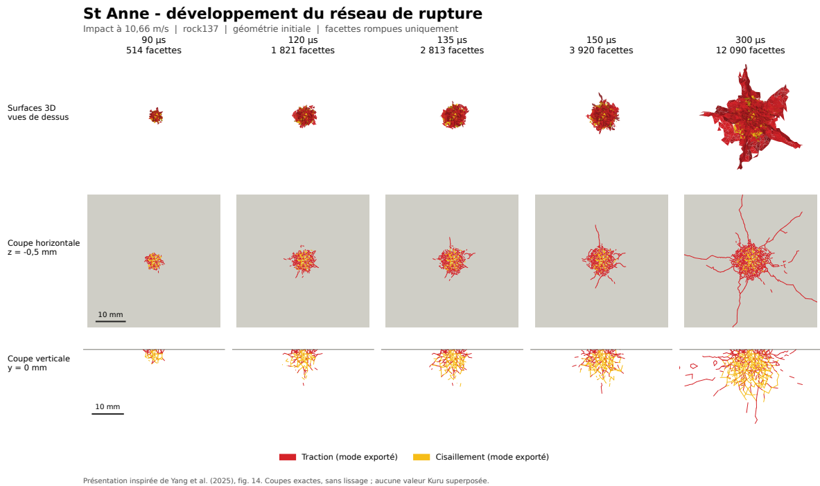
FIGURE 48 – Réplique St Anne : développement du réseau de facettes rompues de 90 à 300 \mu s, vu de dessus, en coupe horizontale à -0,5 mm et en coupe verticale ; couleur selon le mode de rupture.
