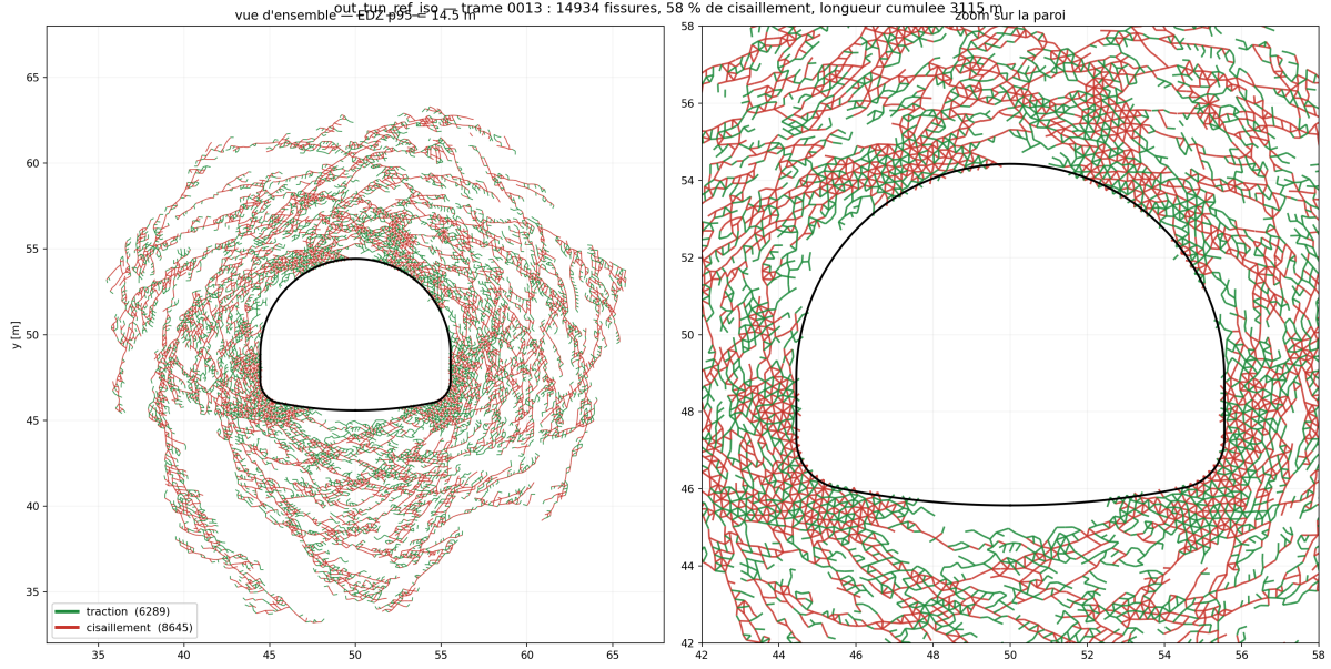
FIGURE 35 – Réseau de fissures du cas de référence, traction en vert et cisaillement en rouge : vue d'ensemble et zoom sur la paroi. L'anneau est quasi circulaire et granulé à l'échelle de l'élément près de la paroi.
