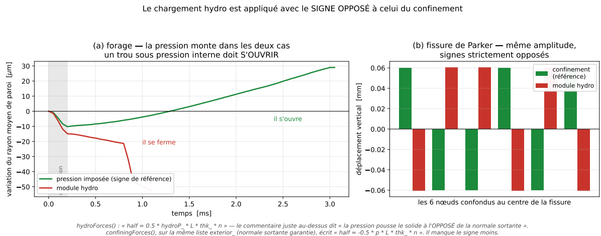
FIGURE 33 – Défaut de signe du 19 août 2026, figure d'archive. (a) La paroi rentre de 50 \mu m sous le module hydraulique et sort de 29 \mu m sous le confinement. (b) Déplacements des six nœuds centraux de la fissure de Parker : même amplitude, signes opposés.
