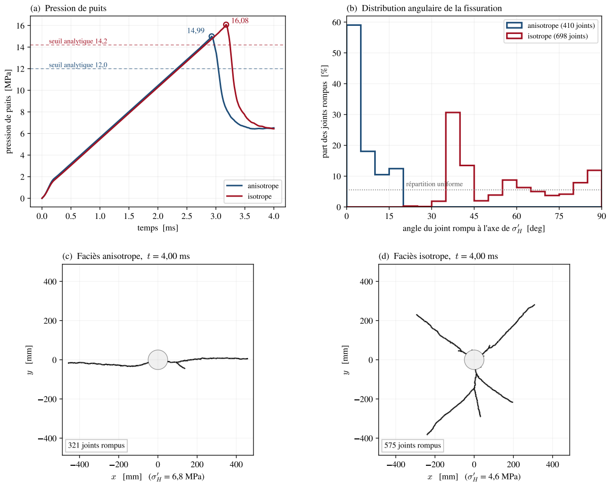
Fracturation hydraulique au forage : effet de l'état de contrainte lointain mêmes maillage, roche, schéma et pompe ; seule \sigma'_H diffère (6,8 contre 4,6 MPa)
