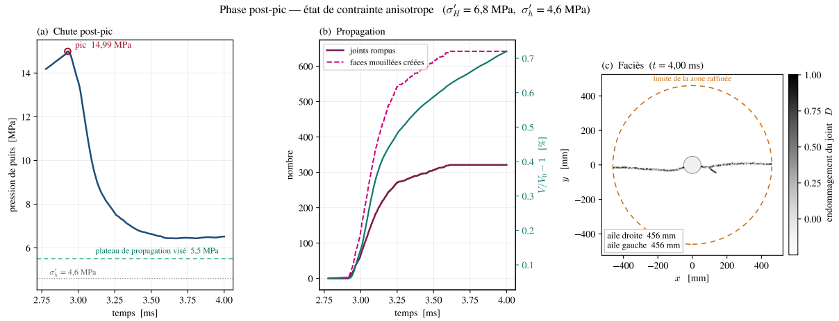
FIGURE 32 – Phase post-pic, état anisotrope : (a) la pression s'infléchit vers 6,5 MPa, au-dessus du plateau de 5,5 MPa de l'article ; (b) joints rompus, faces mouillées et volume de la cavité ; (c) faciès, les ailes atteignant la limite de la zone raffinée.
