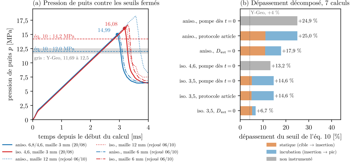
FIGURE 29 – (a) Pression de puits, calculs d'août à 3 mm (traits épais), rejeux du 6 octobre à 12 mm (pointillés) et 6 mm (tirets-points); Hubbert et Willis en tirets, Y-Geo en gris. (b) Dépassement du seuil des sept calculs d'août, statique et incubation.
