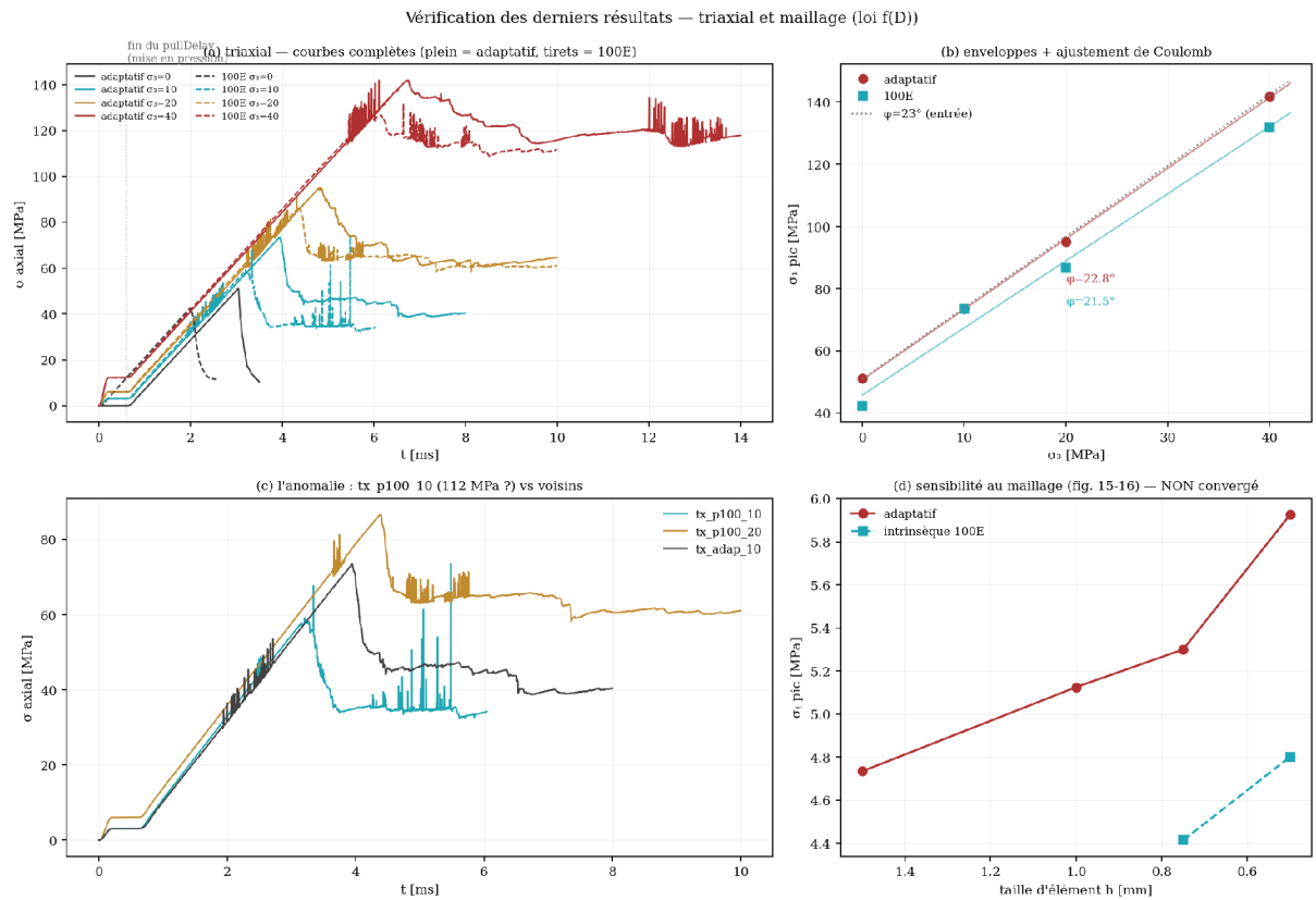
FIGURE 21 – Triaxial 2D et maillage. (a) Courbes axiales, adaptatif et 100E. (b) Ajustement de Coulomb : \varphi = 22,8^\circ et 21,5^\circ (Yan 22,87^\circ et 22,36^\circ ). (c) Courbes à 10 et 20 MPa : oscillations après rupture, cause du pic de 112 MPa enregistré. (d) Pic brésilien selon la maille, adaptatif et 100E.
