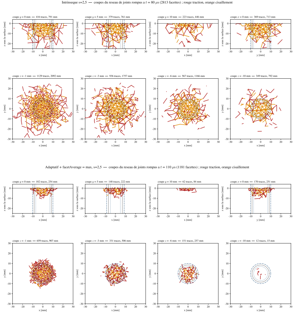
FIGURE 58 – Jumeau grossier de Kuru : traces des joints rompus, insertion intrinsèque à 80 \mu s (haut) et adaptative avec critère du maximum à 110 \mu s (bas).
