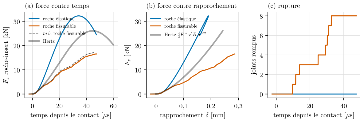
FIGURE 59 – Impact d'un insert en carbure sur roche élastique et fissurable, 50 \mu s, rejoué : force de contact comparée à la solution de Hertz ; le contact maillé est trop raide ; en roche fissurable, amortie, la force baisse avant toute rupture.
