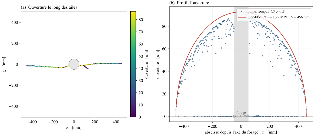
FIGURE 28 – Ouverture des fissures à t = 4 ms, état anisotrope, reconstruite lèvre à lèvre, et ellipse de Sneddon ( \Delta p = 1,92 MPa, L = 456 mm) : 89,0 \mu\text{m} mesurés pour 92,8 \mu\text{m} prédits. Les points à ouverture nulle sont des joints refermés.
