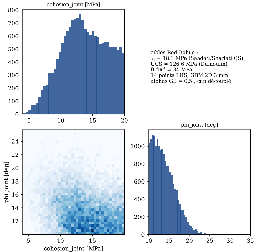
FIGURE 62 – Loi a posteriori de la calibration de juillet, modèle à grains 2D : angle de frottement des joints médian 13,4^\circ , tronqué par la borne a priori; cohésion peu contrainte.
