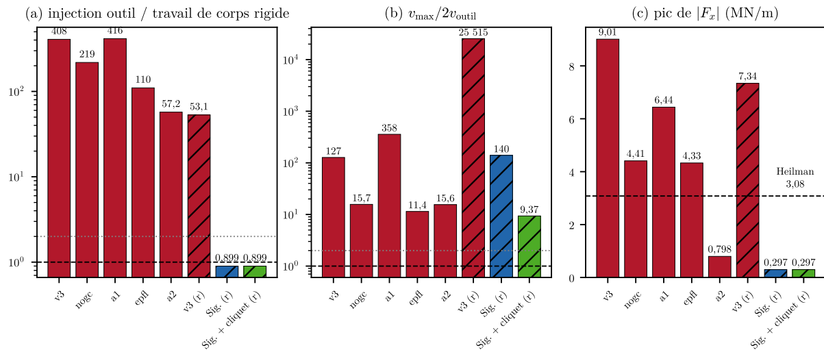
FIGURE 47 – Synthèse des calculs de coupe d’août et du rejeu (r) : (a) rapport d’injection au compteur explicite ; (b) vitesse nodale maximale rapportée à 2v , seuils 1 et 2 ; (c) pic de |F_x| et cible de Heilman.
