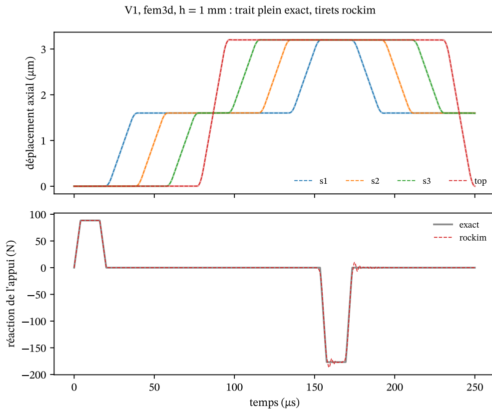
FIGURE 10 – Onde dans une barre, éléments finis 3D, h = 1 mm : déplacements axiaux aux trois stations et au bout libre, et réaction de l'appui, comparés à la série de d'Alembert.
