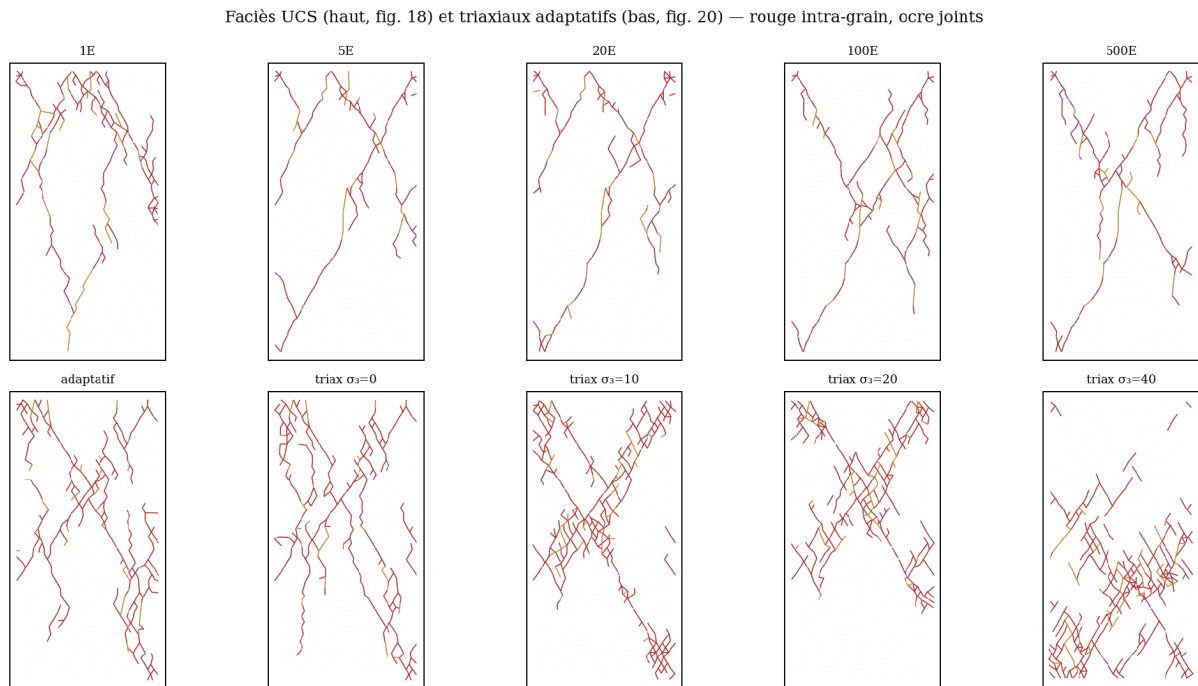
FIGURE 20 – Faciès de compression. Haut : uniaxial intrinsèque de 1E à 500E . Bas : uniaxial adaptatif, puis triaxial adaptatif à 0, 10, 20 et 40 MPa, cisaillement diffus sans fissure traversante à 40 MPa.
