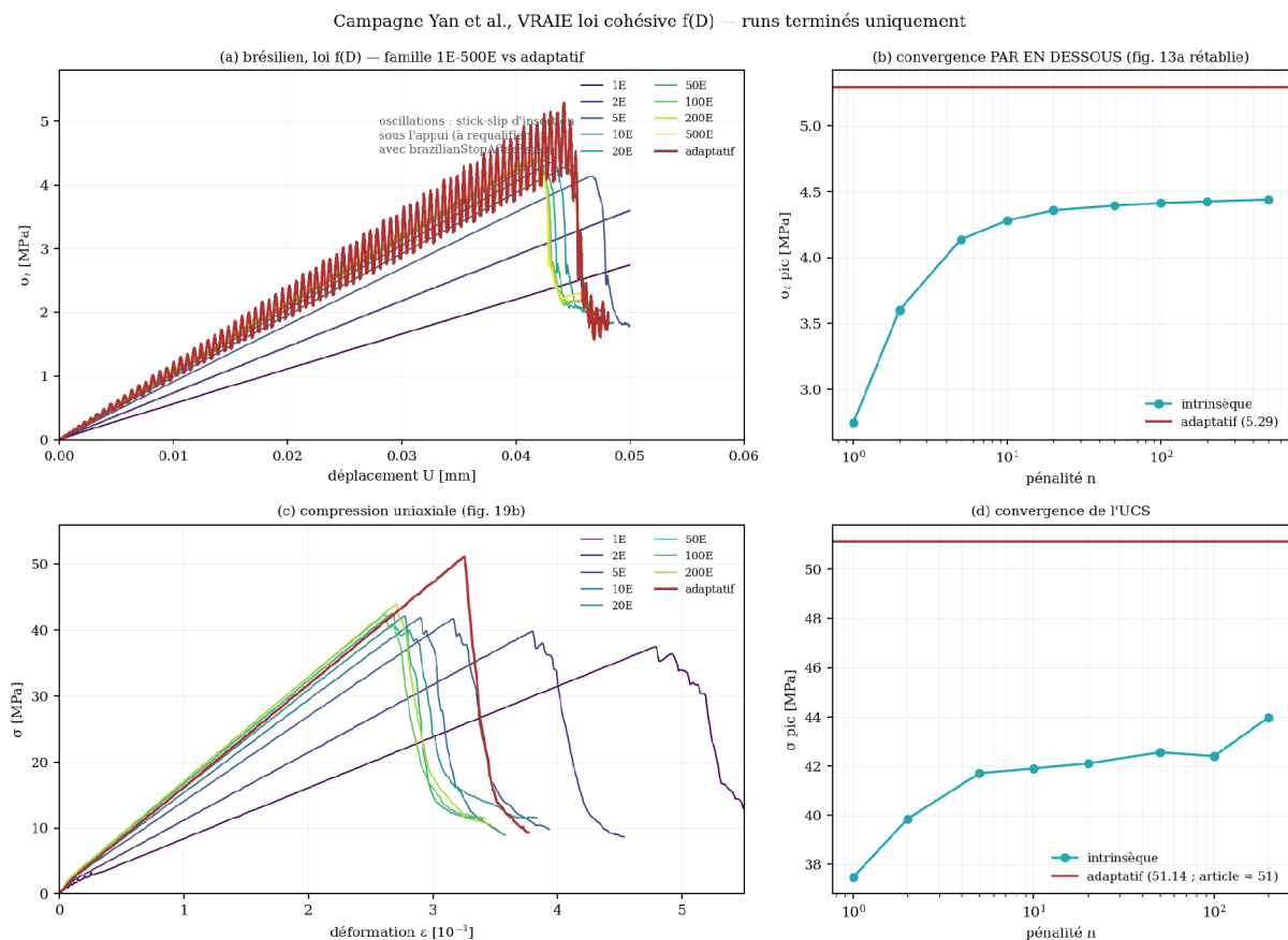
FIGURE 17 – Balayages en pénalité. (a, b) Brésilien : pic croissant de 2,75 à 4,44 MPa, plateau 16 % sous l'adaptatif (5,30 MPa). (c, d) Compression : résistance adaptative 51,1 MPa (Yan environ 51), plateau intrinsèque 44 MPa. La figure affiche 5,29 MPa pour l'adaptatif, les notes d'étude 5,30 MPa.
