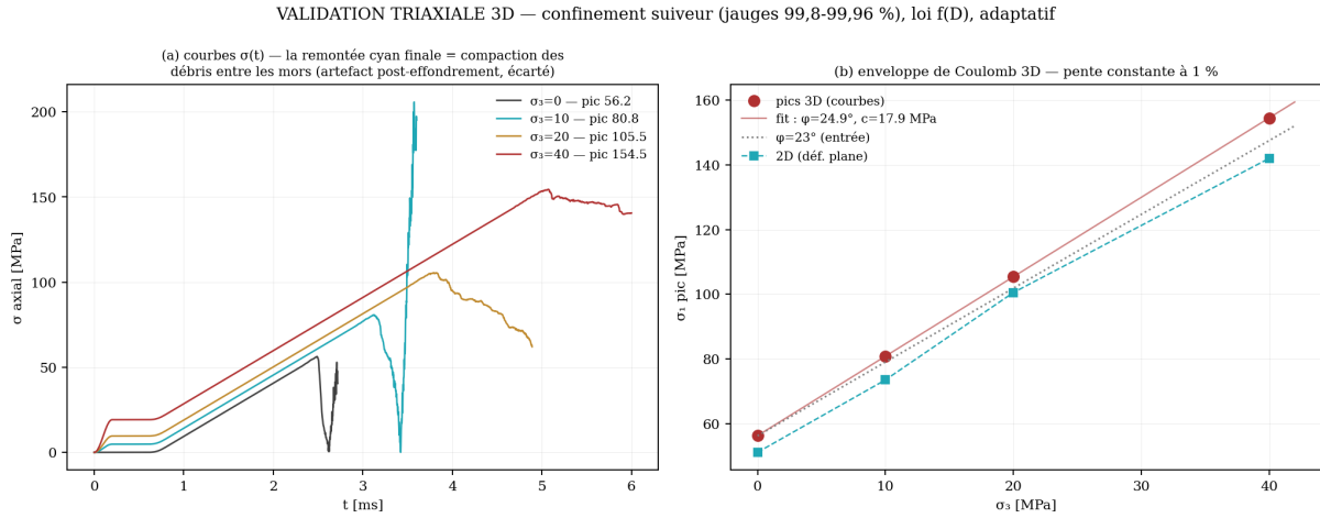
FIGURE 22 – Triaxial 3D adaptatif. (a) Contrainte axiale ; la remontée finale à 10 MPa est une compaction de débris. (b) Enveloppe linéaire, \varphi = 24,9^\circ , c = 17,9 MPa, pour 23^\circ et 16,4 MPa en entrée.
