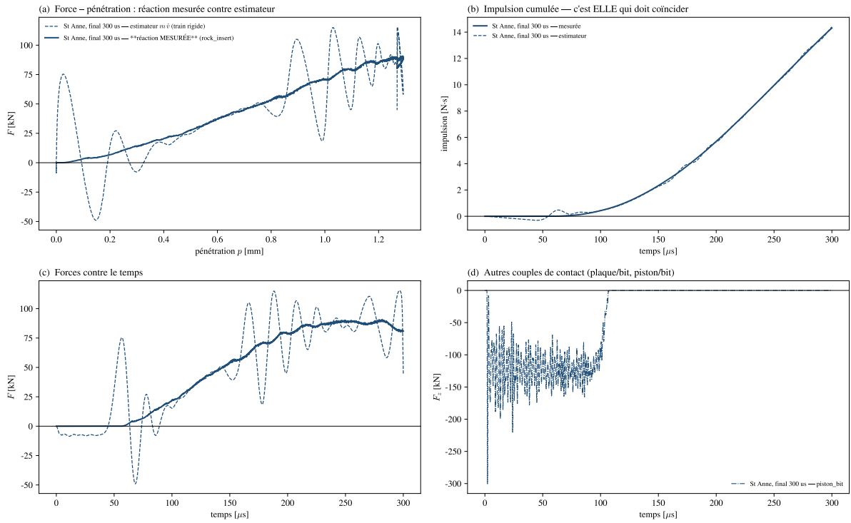
FIGURE 55 – Réplique St Anne : force de contact insert-roche mesurée et estimateur du train rigide, en fonction de la pénétration et du temps, impulsions cumulées et autres paires de contact.
