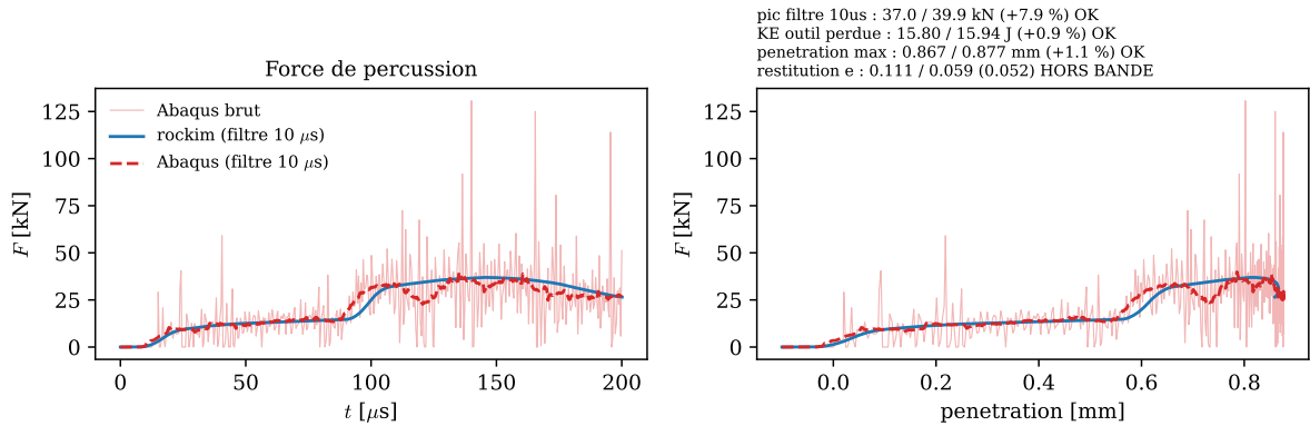
FIGURE 61 – Comparaison de code à code entre rockim et Abaqus/Explicit, loi de Saksala 2011, même maillage : force de percussion filtrée en fonction du temps et de la pénétration.
