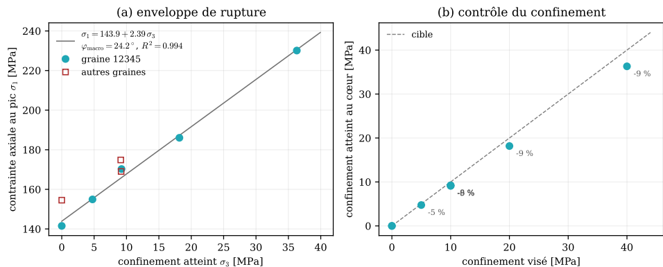
FIGURE 63 – Enveloppe du jeu de juillet. (a) Ajustement de Mohr-Coulomb des pics, angle macroscopique 24,2^\circ . (b) Confinement atteint en fonction du confinement visé, inférieur de 5 à 9 %.
