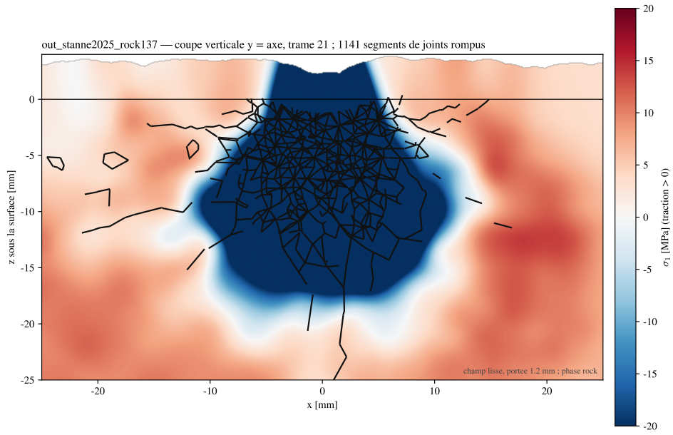
FIGURE 54 – Contrainte principale majeure (traction positive) en coupe verticale par l'axe à 300 \mu s, avec les traces des joints rompus : noyau comprimé sous l'insert, couronne en traction.
