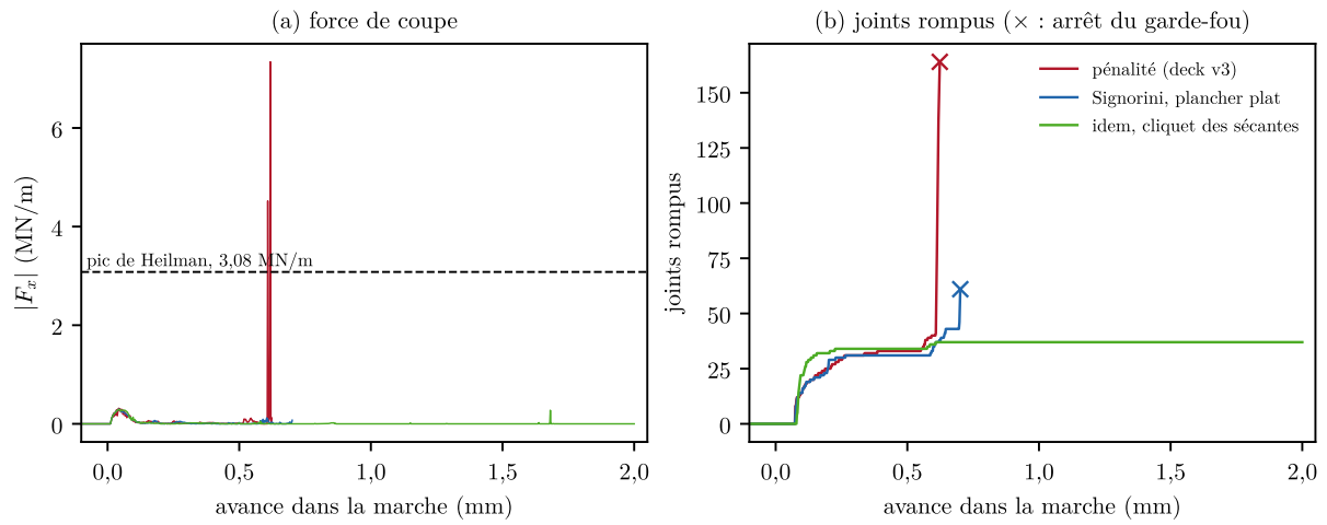
FIGURE 46 – Rejeu du deck v3 : (a) force de coupe |F_x| et pic de Heilman ; (b) joints rompus, en fonction de l’avance de l’arête au-delà de la face d’entaille. Les croix marquent l’arrêt par le garde-fou d’énergie.
