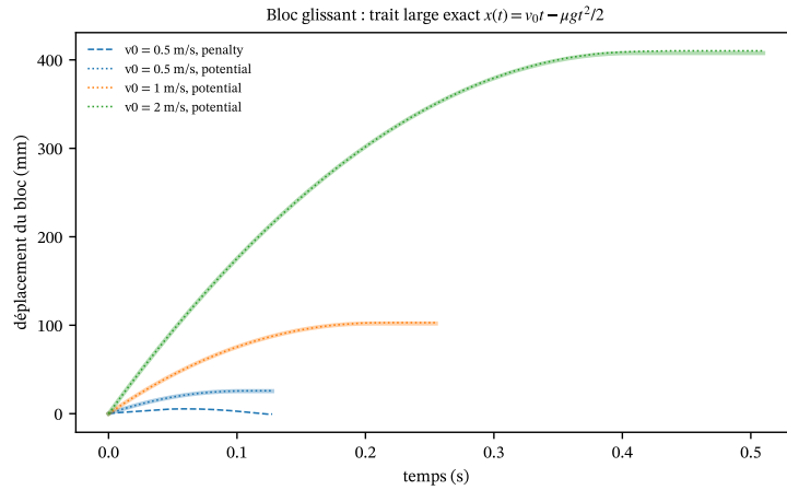
FIGURE 13 – Bloc glissant : déplacement en fonction du temps pour trois vitesses initiales, contact par potentiel et par pénalité nœud-face, solution exacte en trait large.
