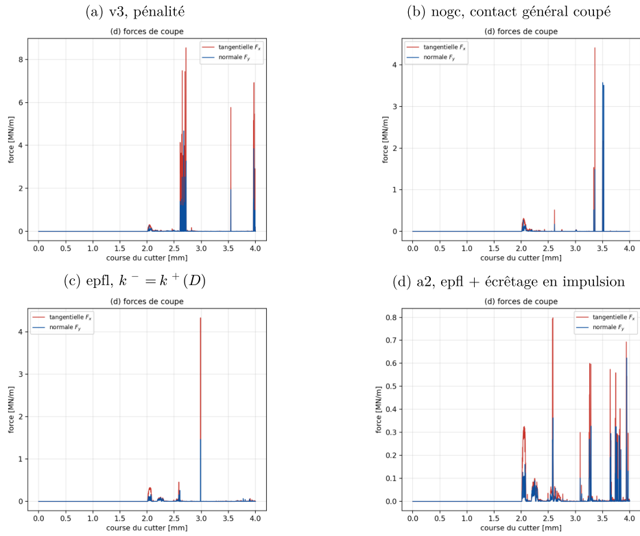
FIGURE 45 – Forces de coupe tangentielle (rouge) et normale (bleu) en fonction de la course, calculs d'août 2026, planches d'archive recadrées : (a) v3 ; (b) contact général coupé ; (c) pénalité de compression de Ghesquière-Diérckx et al. ; (d) même pénalité et écrêtage en impulsion.
