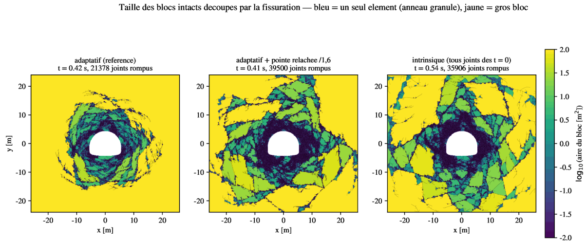
FIGURE 39 – Taille des blocs intacts (aire en échelle logarithmique) pour l'insertion adaptative, l'adaptative avec k_{\text{tip}} = 1,6 et l'intrinsèque : l'adaptative granule un anneau, les deux autres découpent des blocs polygonaux de quelques dizaines à quelques centaines de m 2 .
