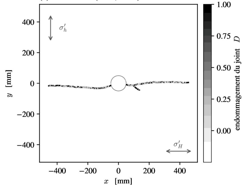
(d) Fissuration ( t = 4,00 ms)
