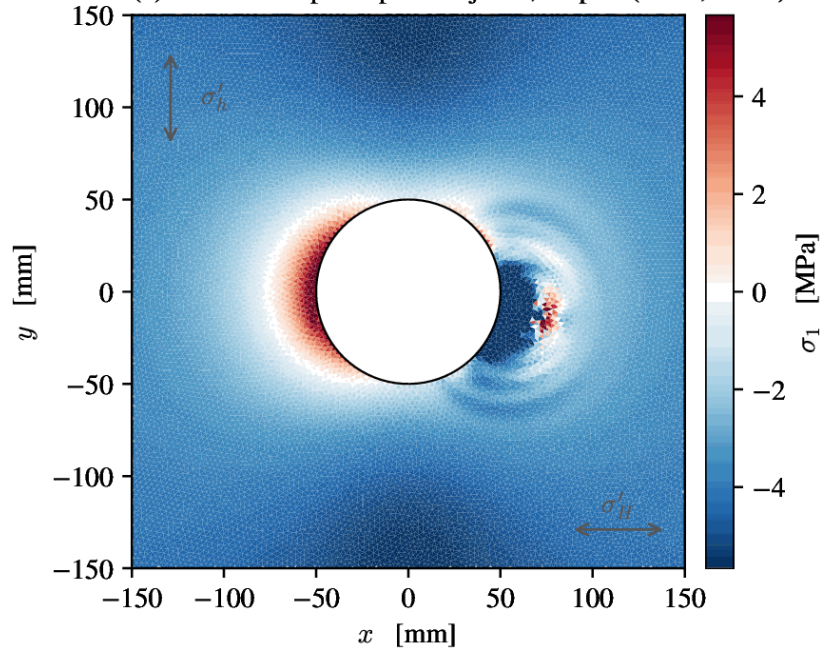
(c) Contrainte principale majeure, au pic ( t = 2,93 ms)
