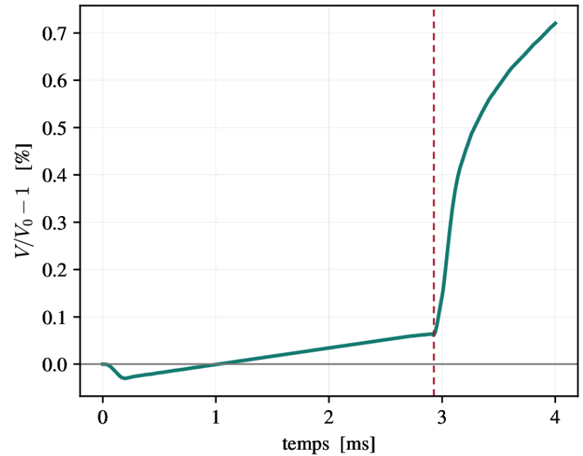
(b) Volume de la cavité
