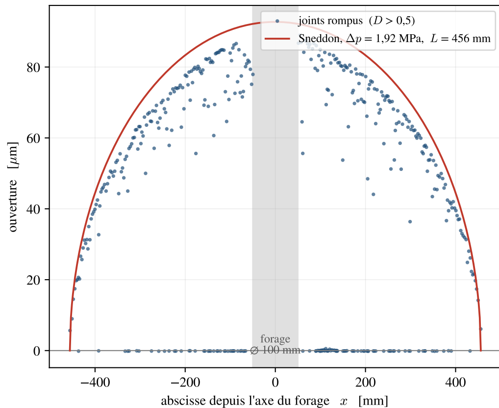
(b) Profil d'ouverture
