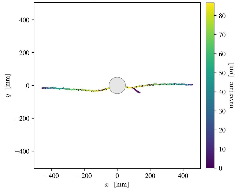
(a) Ouverture le long des ailes
