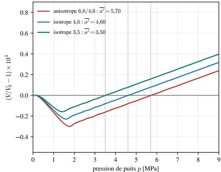
(a) La cavité retrouve son volume initial quand p atteint \overline{\sigma'}
