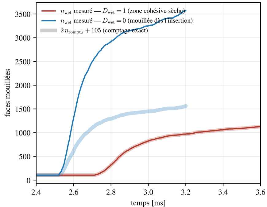
(b) Le front mouillé : chaque joint rompu livre ses deux lèvres
