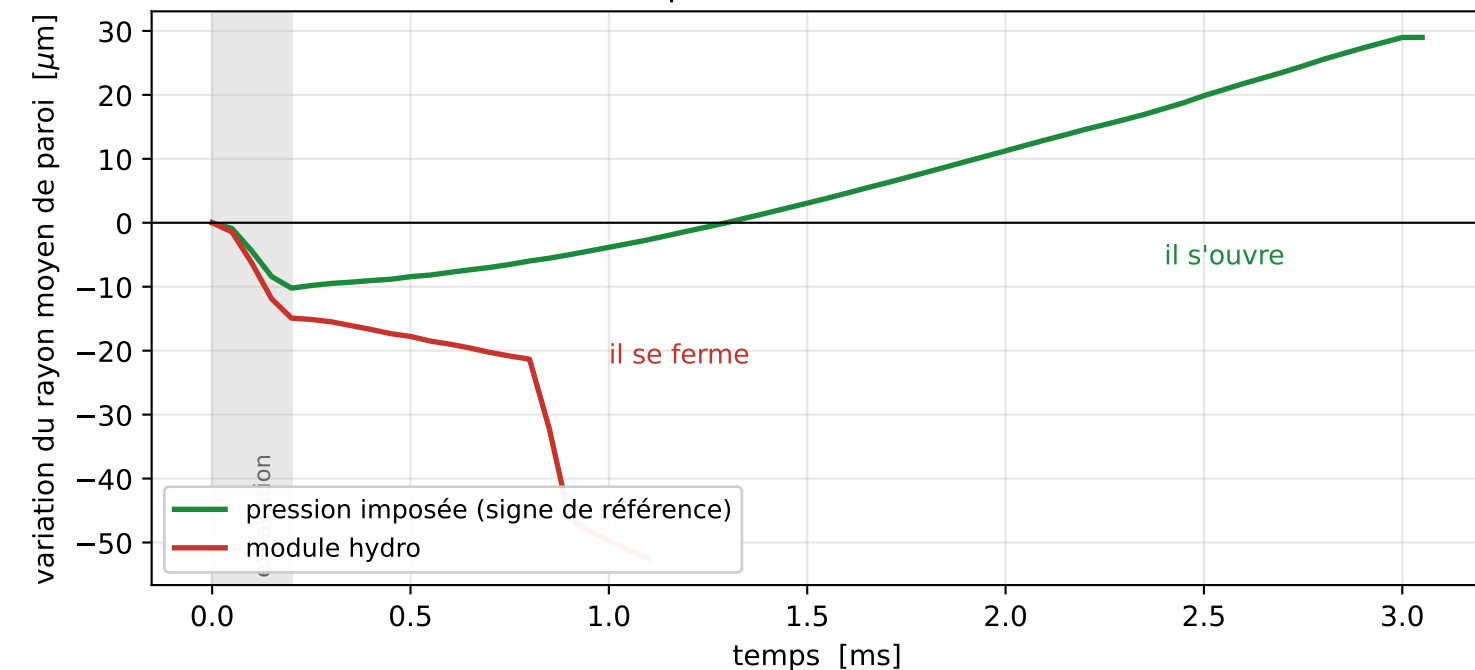
(a) forage — la pression monte dans les deux cas un trou sous pression interne doit S'OUVRIR
