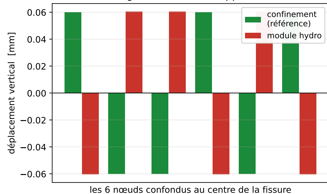
(b) fissure de Parker — même amplitude, signes strictement opposés
