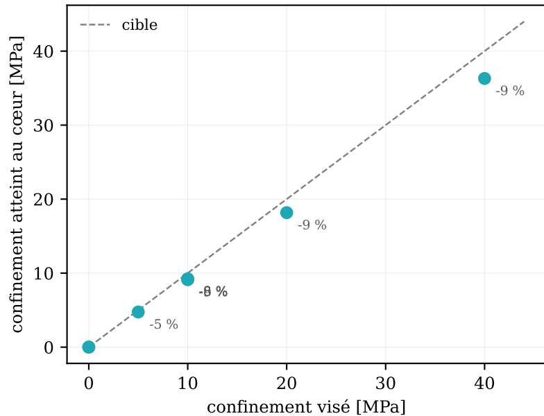
(b) contrôle du confinement
