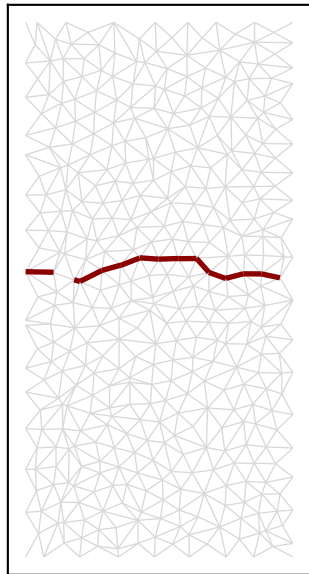
fissure finale (joints rompus)
