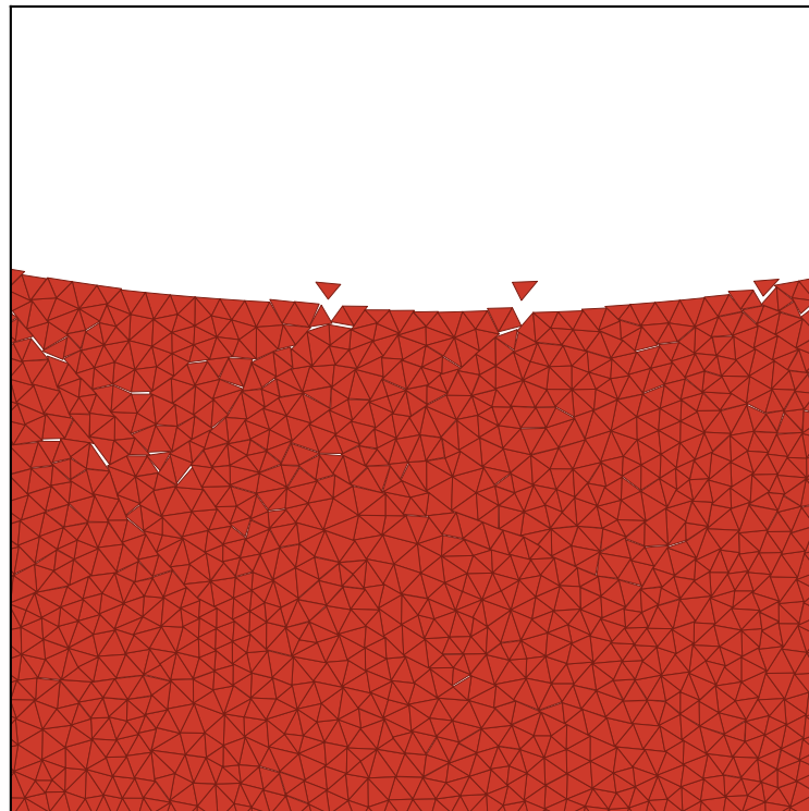
Soulèvement du radier
