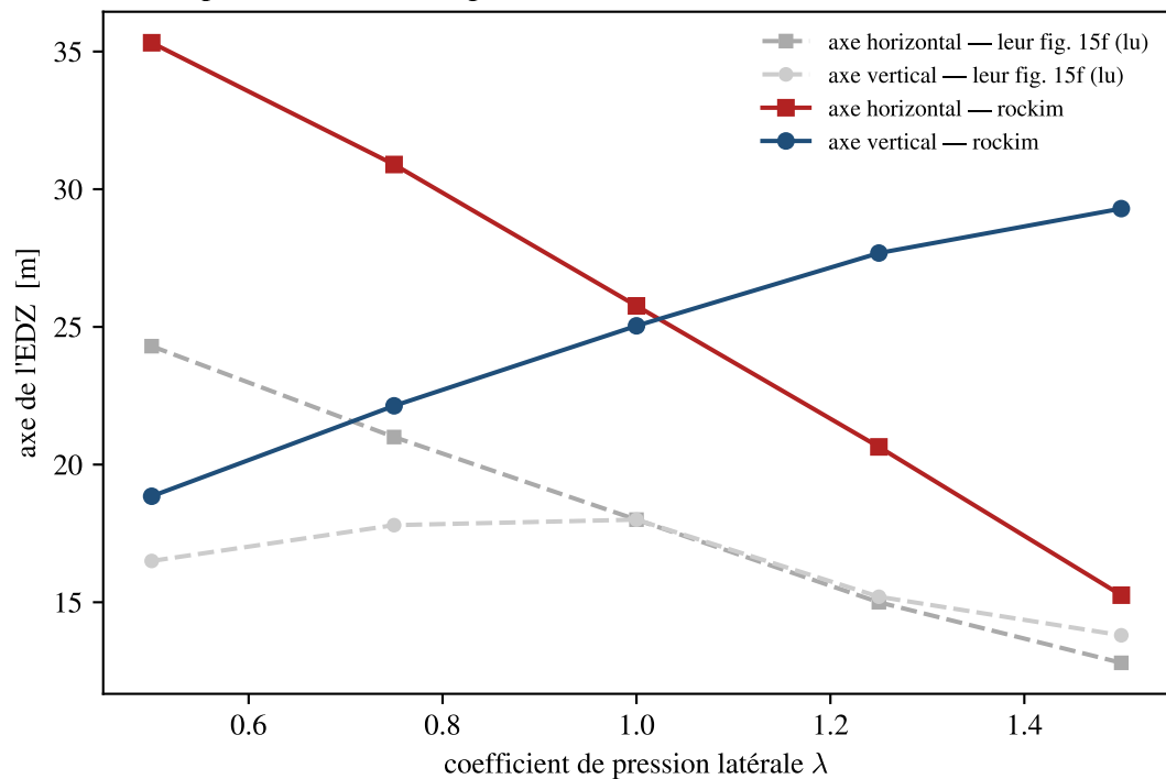
(a) Ellipse de l'EDZ (leur fig. 15f)
