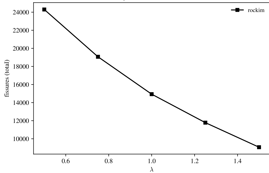
(b) Nombre de fissures (leur fig. 16a : décroissant)
