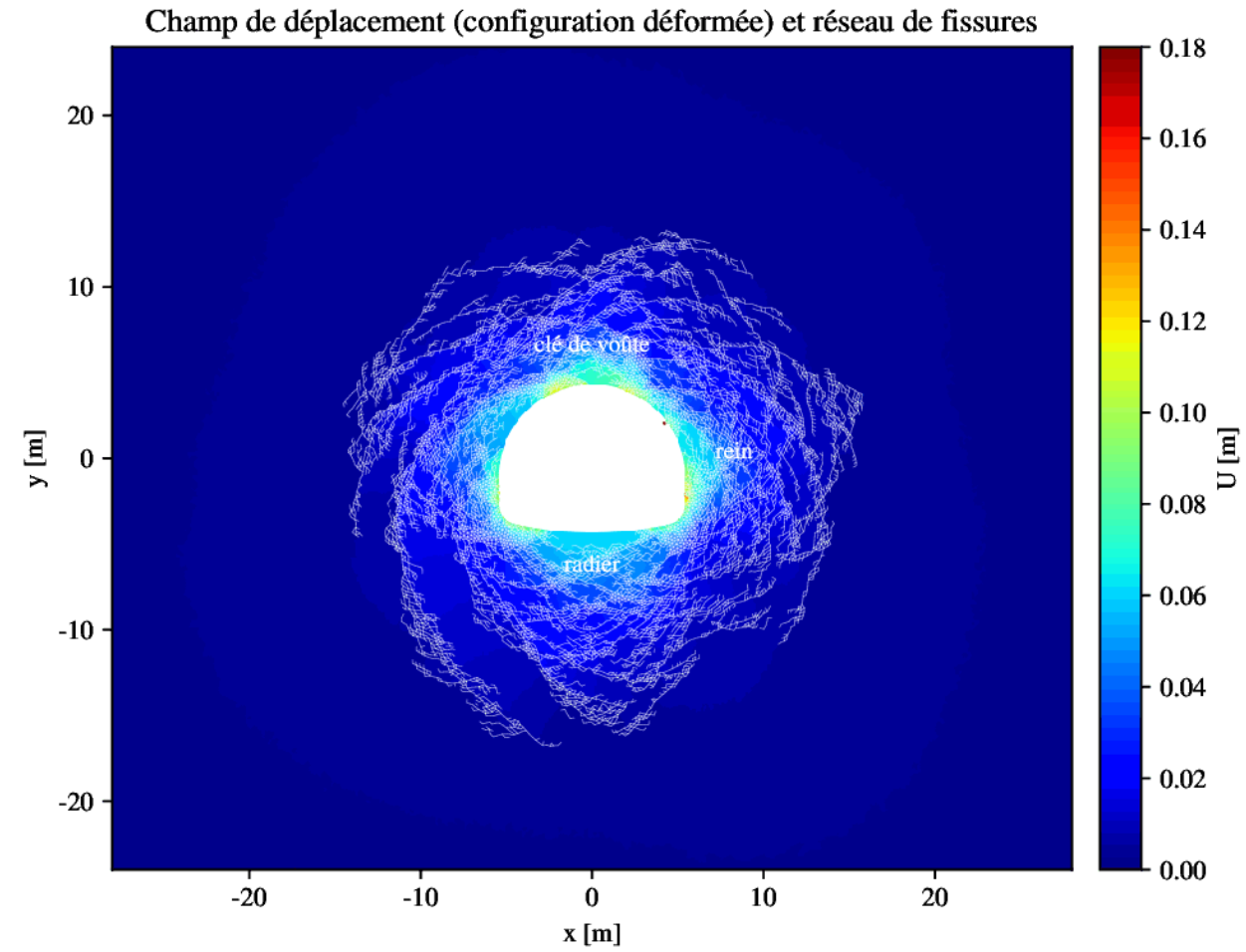
Compression-cisaillement
