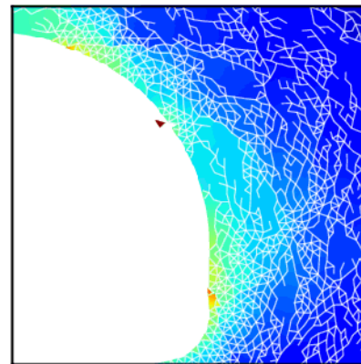
Compression-cisaillement
