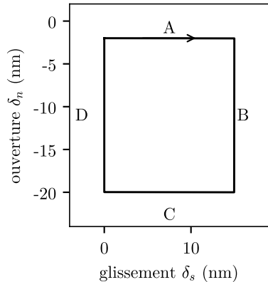
(a) trajet imposé, cycle intact
