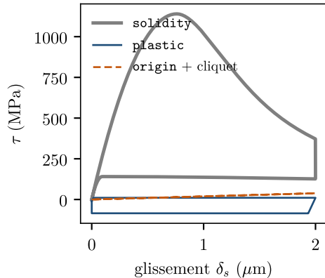
(c) cycle endommagé, D_{\max} 0,47 à 0,88
