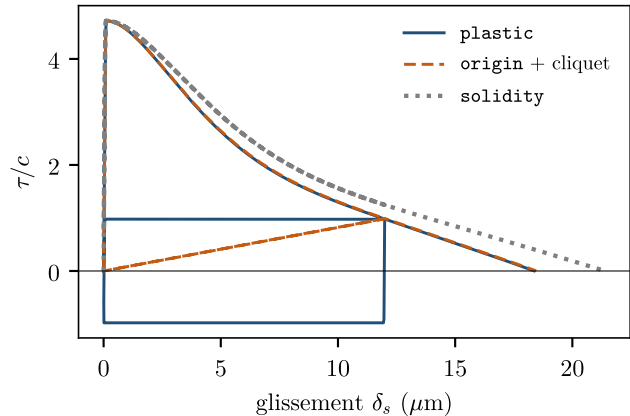
(b) cisaillement sous \sigma_n = -60 \text{ MPa} , décharge à 12 \mu\text{m}
