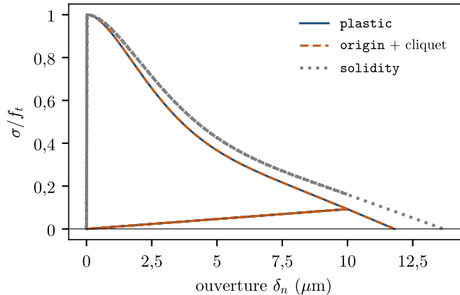
(a) traction, décharge à 10 \mu\text{m}
