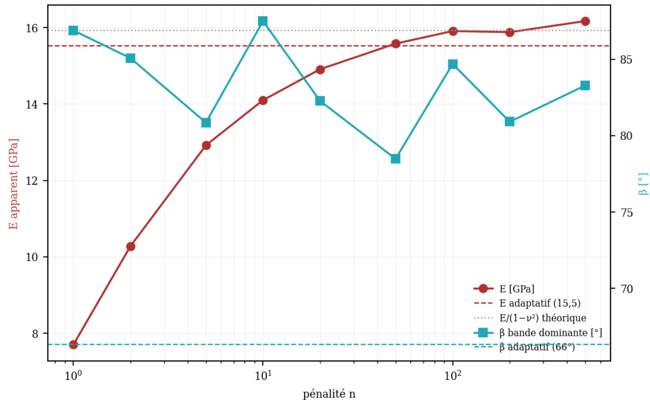
Fig. 19a — module apparent et angle de rupture vs pénalité
