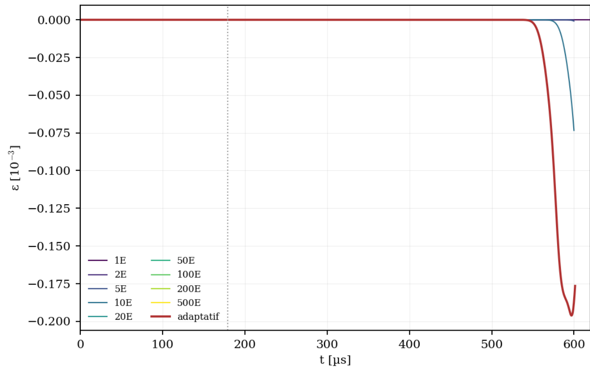
(b) jauge M2 — onde transmise
