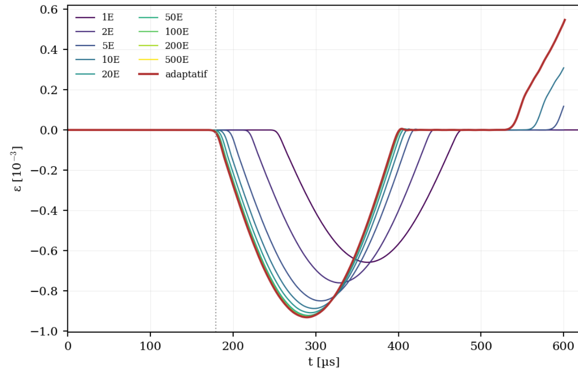
(a) jauge M1 — onde incidente (+ réfléchi)
