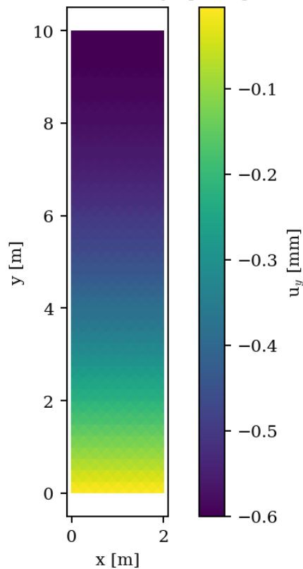
(a) bande pesante adaptative — u_y (fig. 8) tête : -0,601 mm = analytique (équ. 20)
