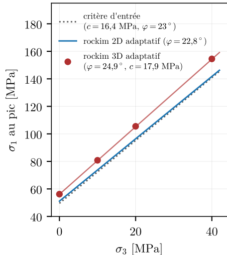
(a) enveloppe de Coulomb
