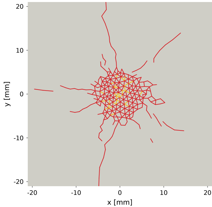
(a) Surface initiale : z = 0 430 arêtes uniques débouchantes
