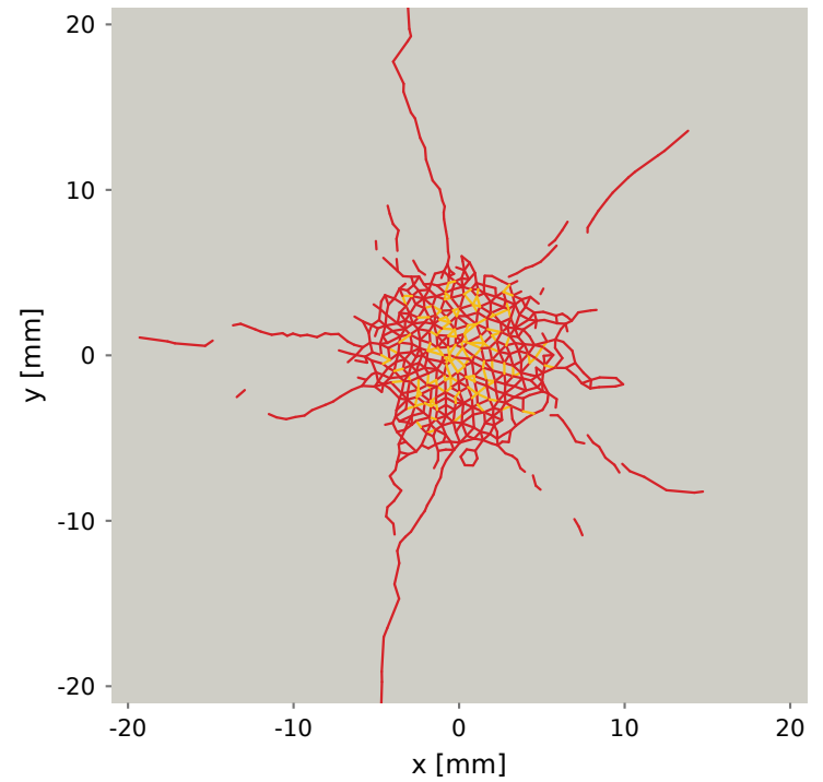
(b) Coupe sous la surface : z = -0,5 mm 982 segments d'intersection
