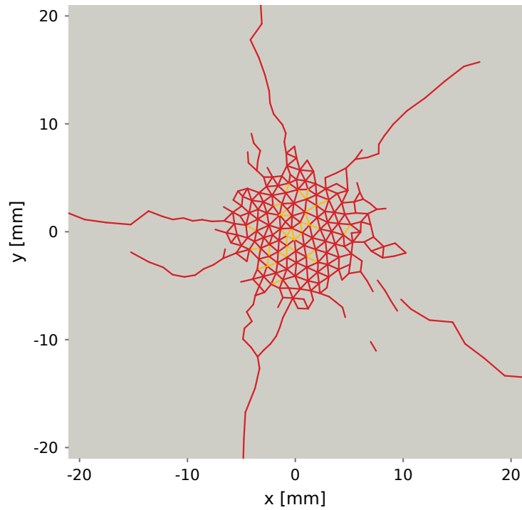
(a) Surface initiale : z = 0 491 arêtes uniques débouchantes
