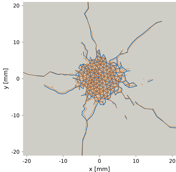
(c) Superposition dans la géométrie initiale Bleu : surface ; orange : coupe à -0,5 mm
