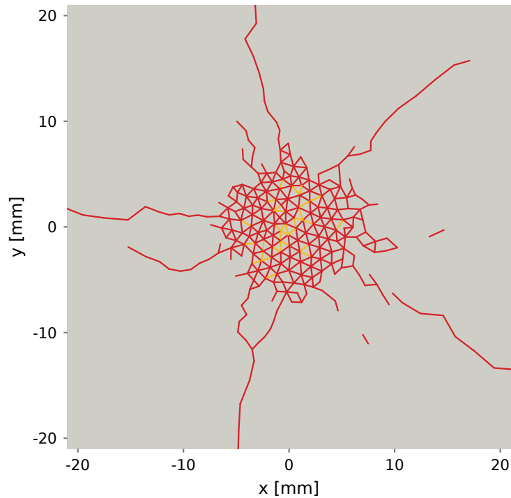
(a) Surface initiale : z = 0 496 arêtes uniques débouchantes
