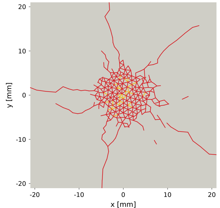
(d) Mêmes arêtes de surface, positions courantes Projection XY ; ce n'est pas une coupe à z = 0
