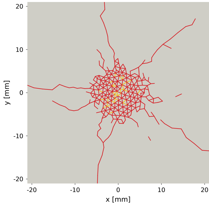
(a) Surface initiale : z = 0 503 arêtes uniques débouchantes
