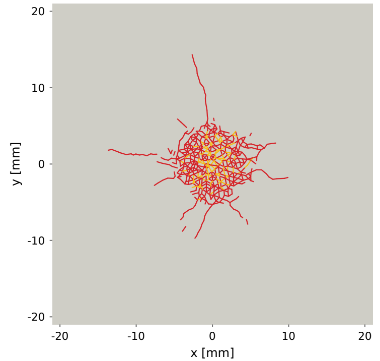
(b) Coupe sous la surface : z = -0,5 mm 700 segments d'intersection
