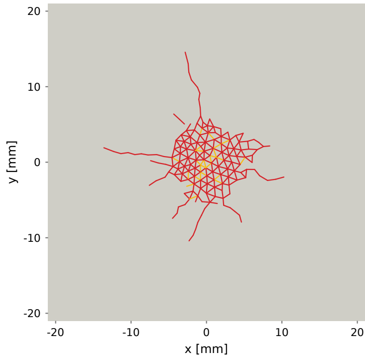
(a) Surface initiale : z = 0 301 arêtes uniques débouchantes
