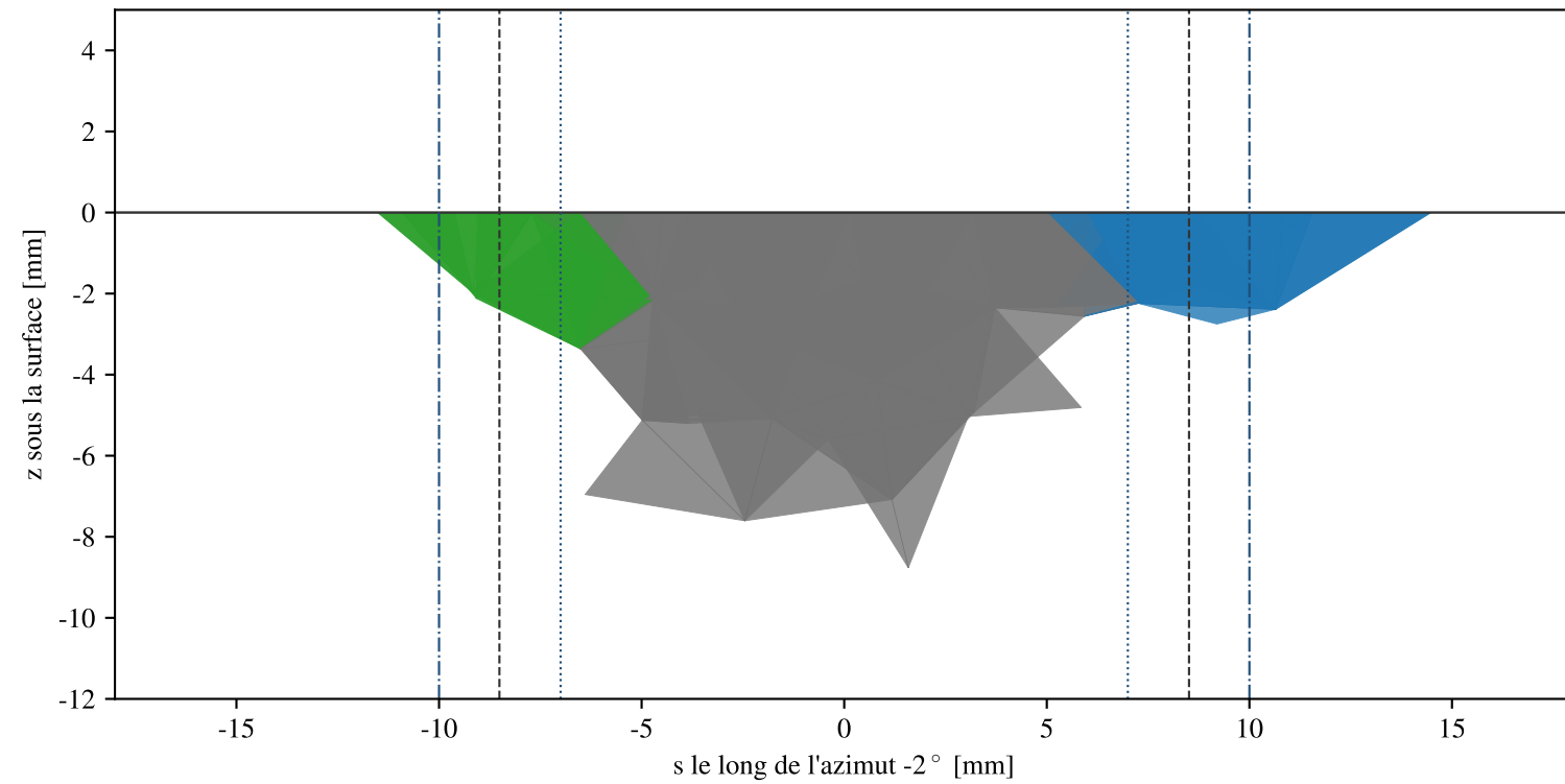
(b) coupe verticale par l'axe et la pointe radiale, |d| < 1.5 \text{ mm}
