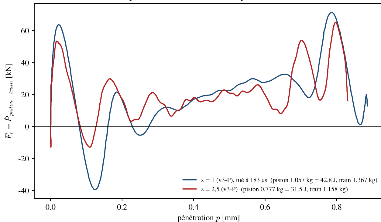
(a) Réaction de la roche (quantité de mouvement) contre pénétration
