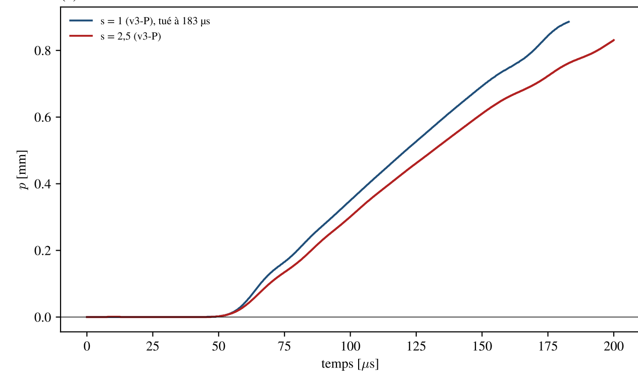
(d) Pénétration de l'insert
