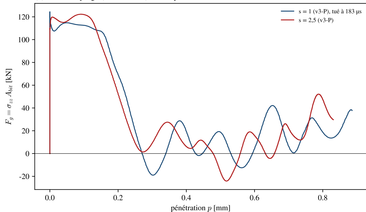
(b) Force de jauge (mi-bit, onde) contre pénétration
