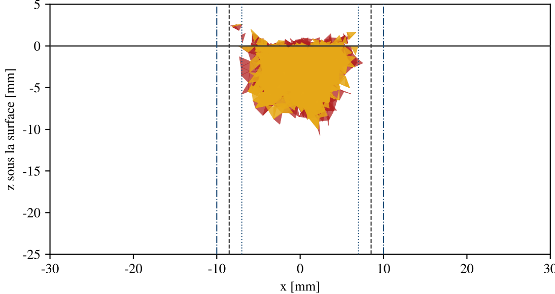
(c) Coupe |y| < 5 mm, par mode
