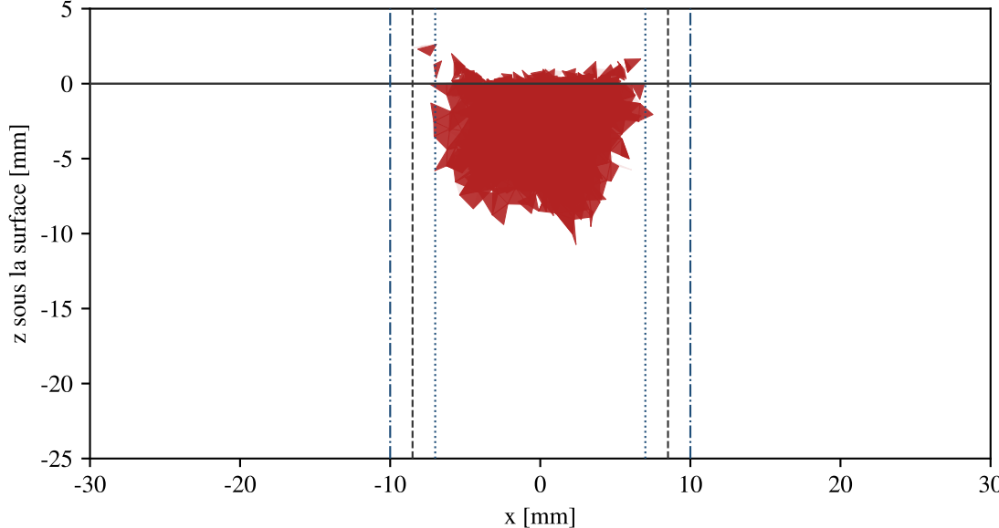
(f) Coupe |y| < 5 mm — fissures / broye
