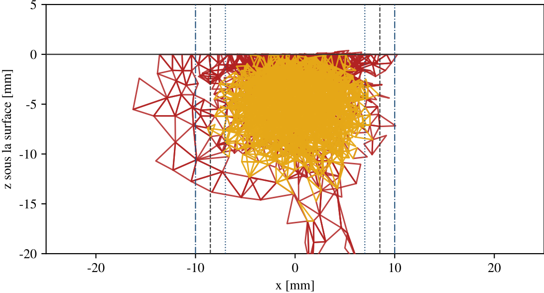
(c) Coupe |y| < 5 mm, par mode
