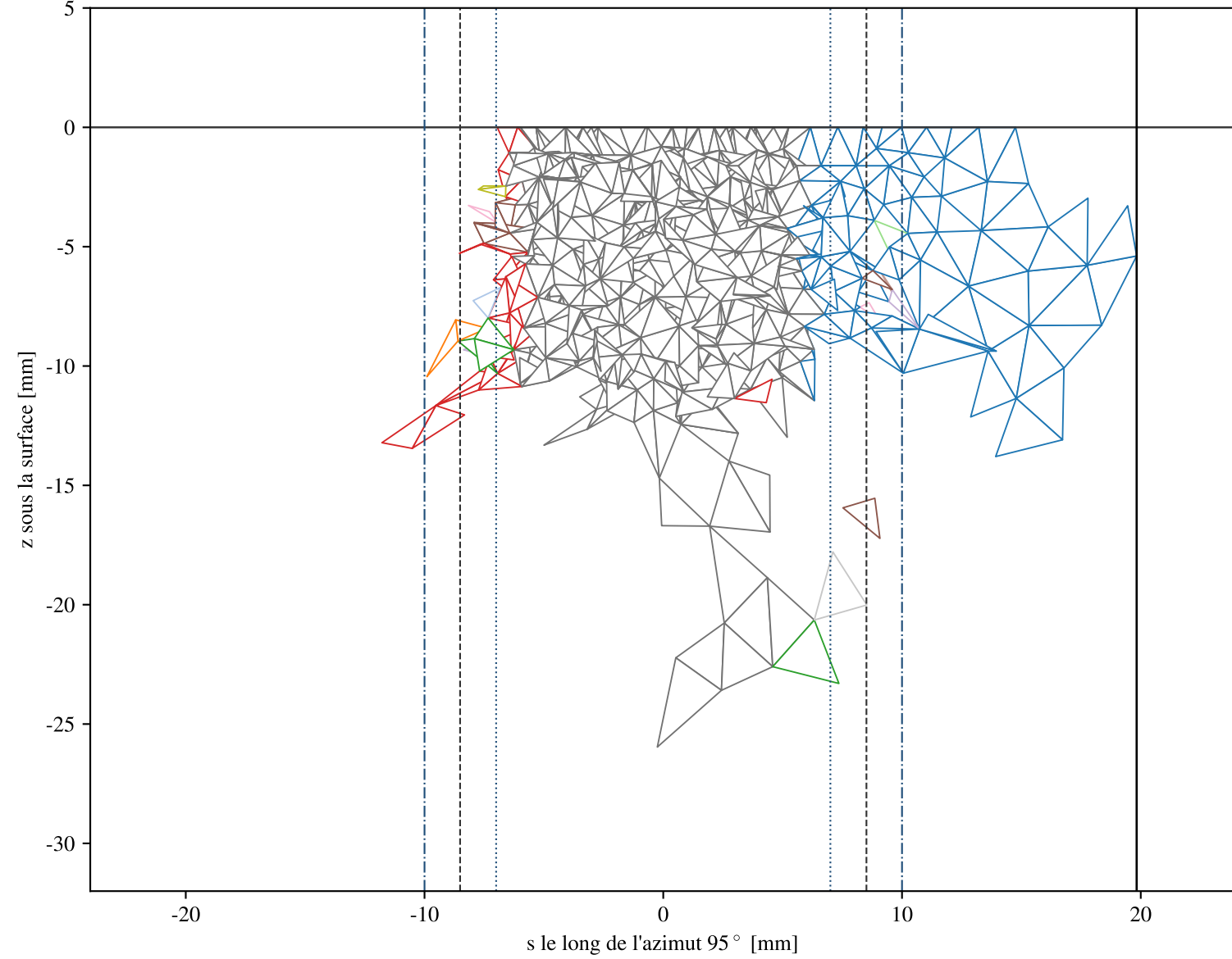
(b) coupe verticale par l'axe et la pointe radiale, |d| < 1.5 \text{ mm}
