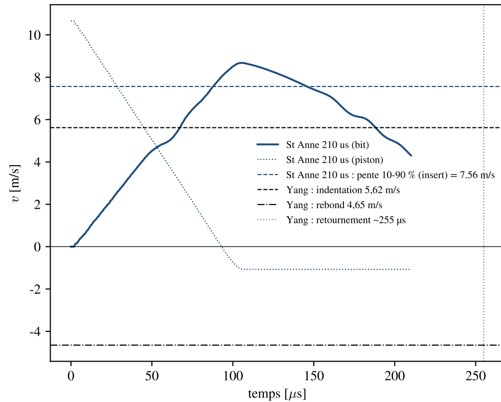
(b) Vitesse du bit et du piston, vers le bas &gt; 0
