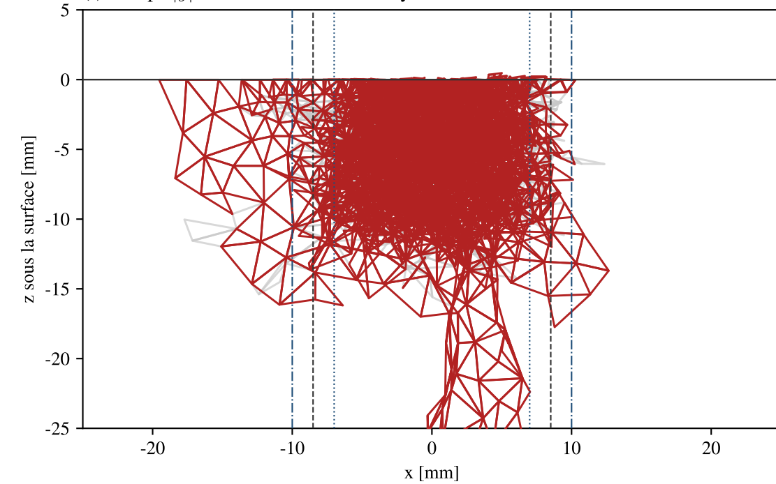
(f) Coupe |y| < 5\ \text{mm} — fissures / broye
