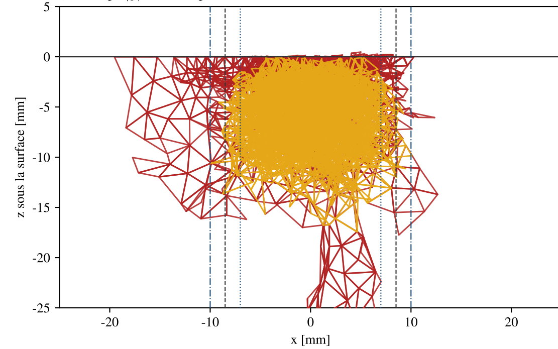
(c) Coupe |y| < 5\ \text{mm} , par mode
