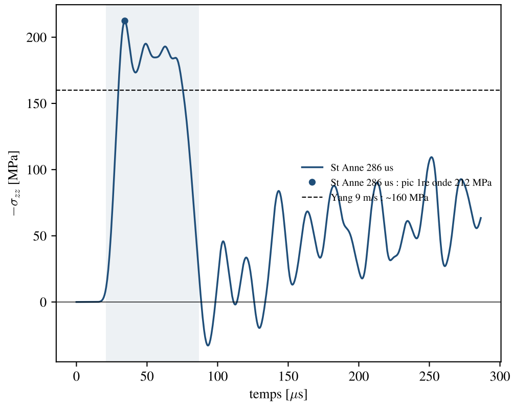
(a) Contrainte de jauge à mi-bit (leur fig. 8-9a)
