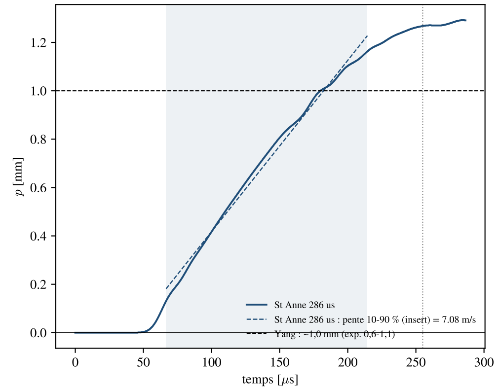
(c) Enfoncement de l'insert (leur fig. 8-9b)
