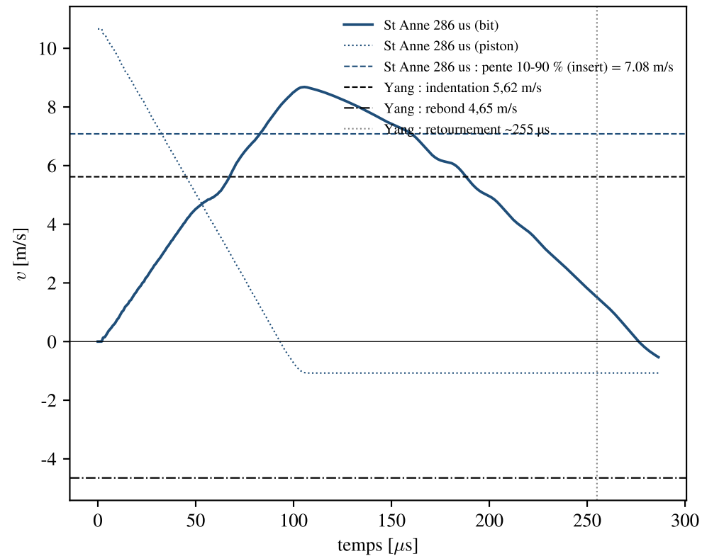
(b) Vitesse du bit et du piston, vers le bas &gt; 0
