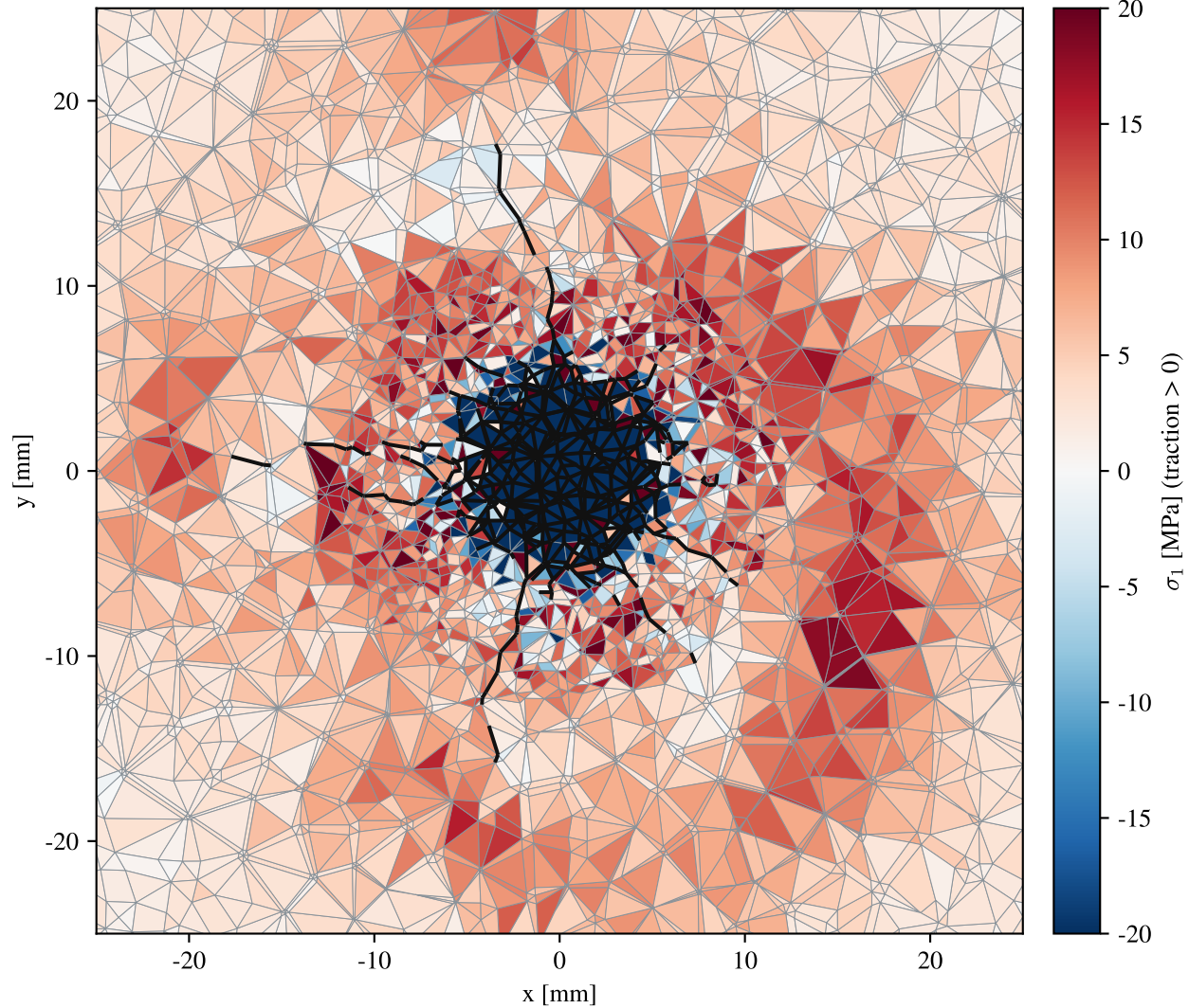
out_stanne2025_rock137 — vue de dessus, z = -2.0 mm, trame 12 ; 876 segments de joints rompus
