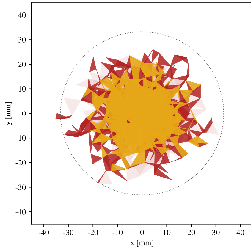
(c) Fissures, vue de dessus ( t = 80 \mu s)
