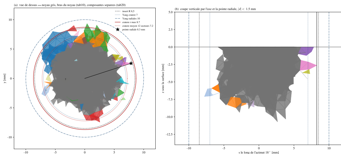
FIGURE 54 – Réplique Kuru, maillage fin, à 180 \mu s : réseau connecté vu de dessus et en coupe ; noyau dense de 7 à 9 mm, pas d'étoile radiale.
