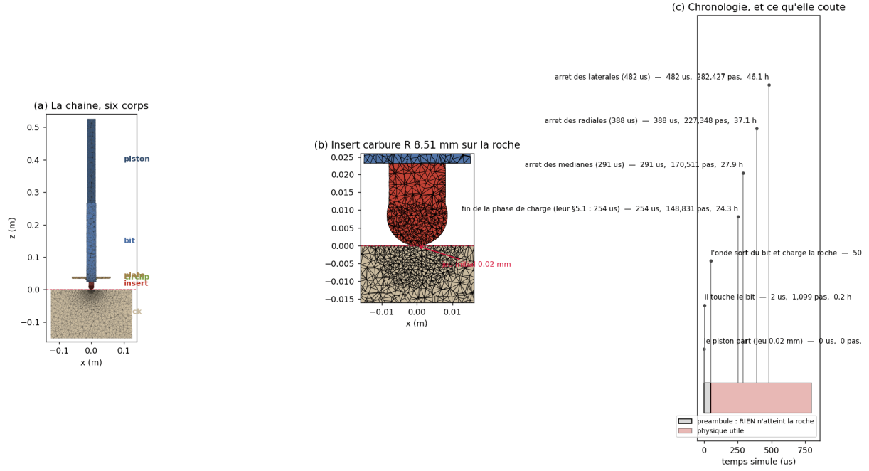
FIGURE 45 – Montage de la réplique St Anne : chaîne de six corps, insert en carbure posé à 0,02 mm de la roche, et coût en temps de calcul des événements de la chronologie.
