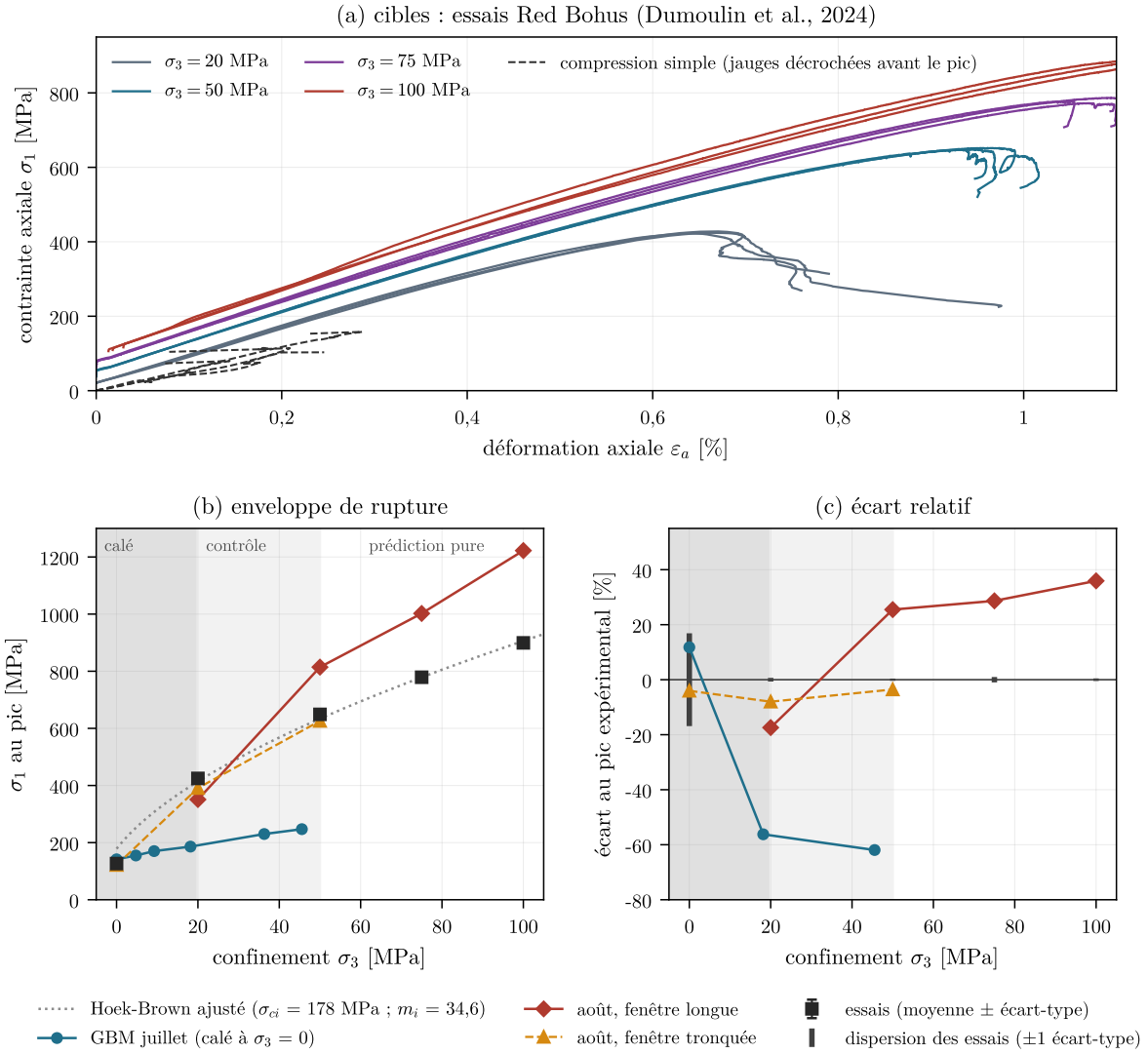
FIGURE 61 – Calibration Red Bohus. (a) Essais de Dumoulin et al. (b) Enveloppe : le jeu de juillet sous-estime le confinement, celui d’août le surestime au-delà d’environ 35 MPa. (c) Écart au pic expérimental.
