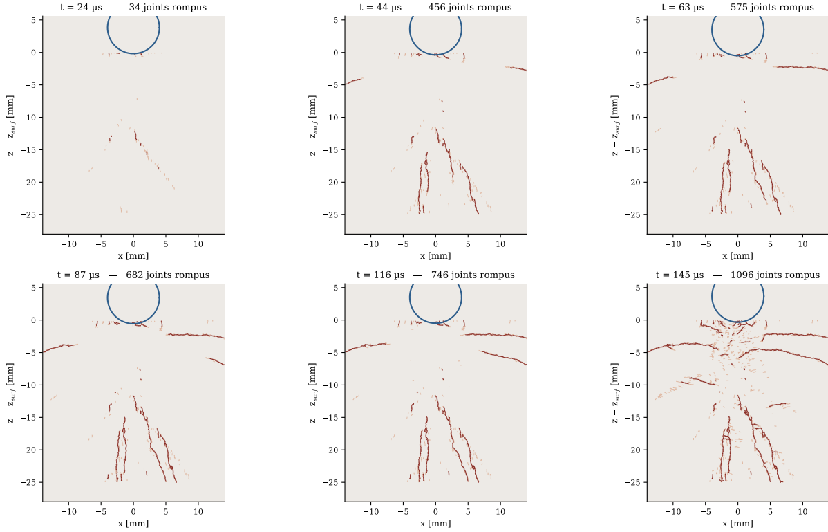
Développement des fissures — indentation 2D, modèle de Yan, maille 0,15 mm
