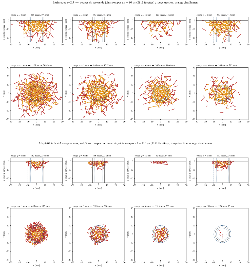
FIGURE 55 – Jumeau grossier de Kuru : traces des joints rompus, insertion intrinsèque à 80 \mu s (haut) et adaptative avec critère du maximum à 110 \mu s (bas).
