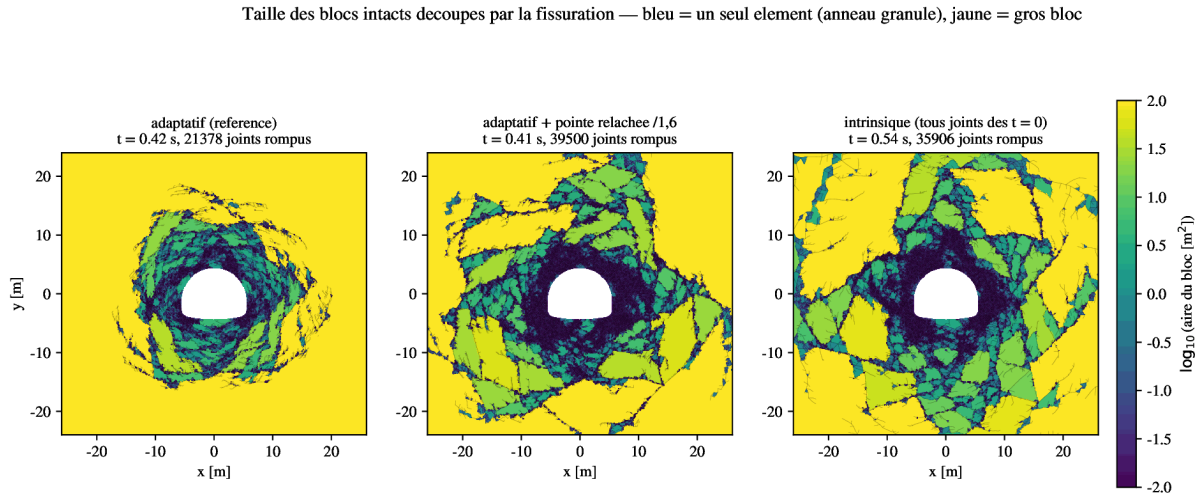
FIGURE 39 – Taille des blocs intacts (aire en échelle logarithmique) pour l'insertion adaptative, l'adaptative avec k_{tip} = 1,6 et l'intrinsèque : l'adaptative granule un anneau, les deux autres découpent des blocs polygonaux de quelques dizaines à quelques centaines de m 2 .
