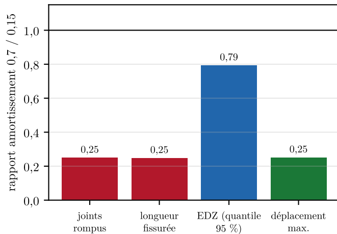
(d) effet de l'amortissement local, maillage d'essai
