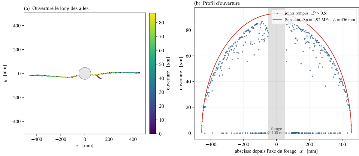
Ouverture des fissures — état de contrainte anisotrope ( t = 4,00 ms, p = 6,52 MPa)
