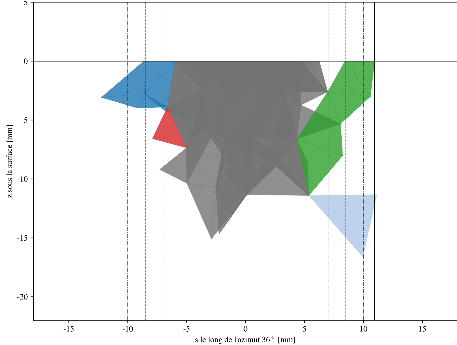
(b) coupe verticale par l'axe et la pointe radiale, |d| < 1.5 \text{ mm}
