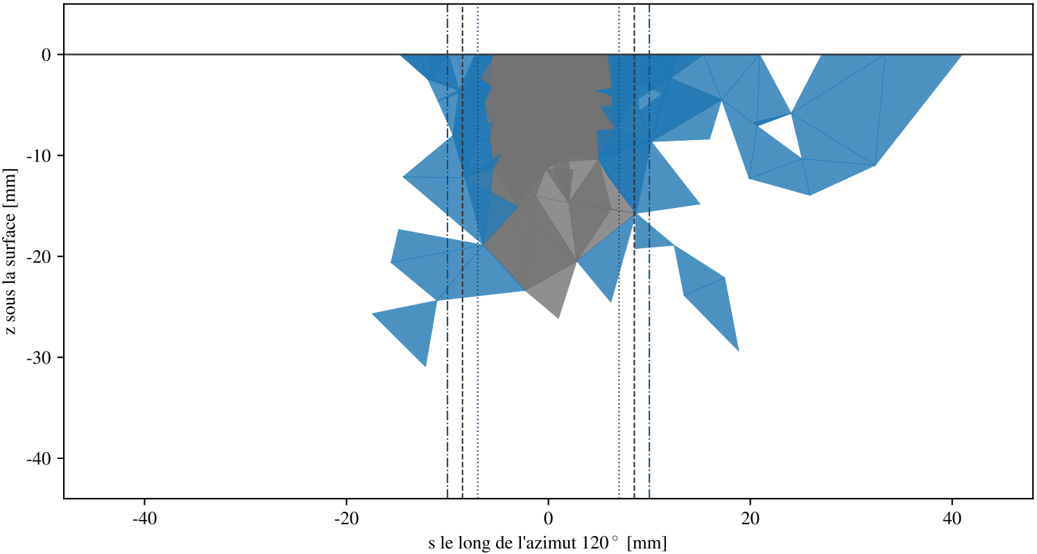
(b) coupe verticale par l'axe et la pointe radiale, |d| < 1.5 mm
