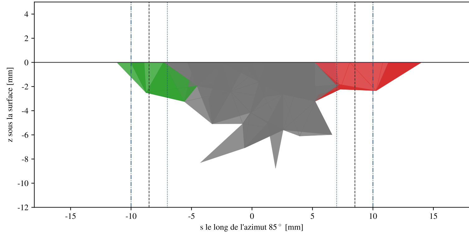
(b) coupe verticale par l'axe et la pointe radiale, |d| < 1.5 mm
