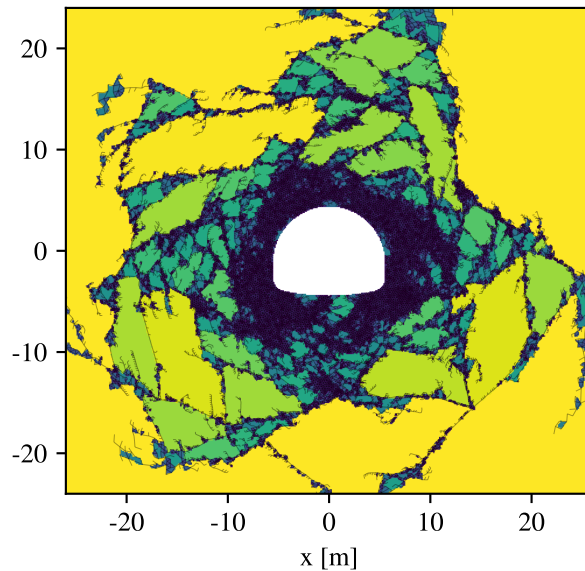
adaptatif + pointe relachee /1,6 t = 0.41 s, 39500 joints rompus
