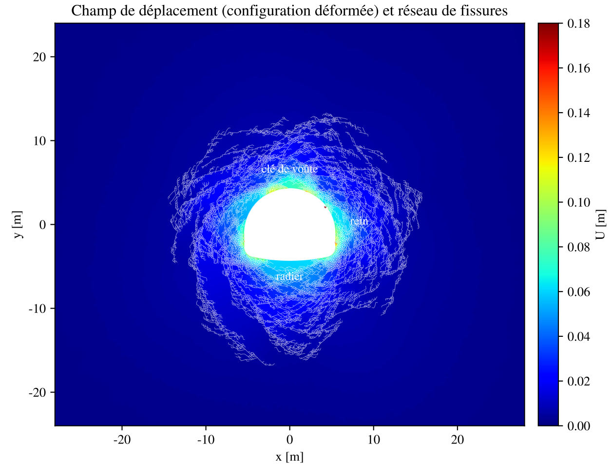
Compression-cisaillement
