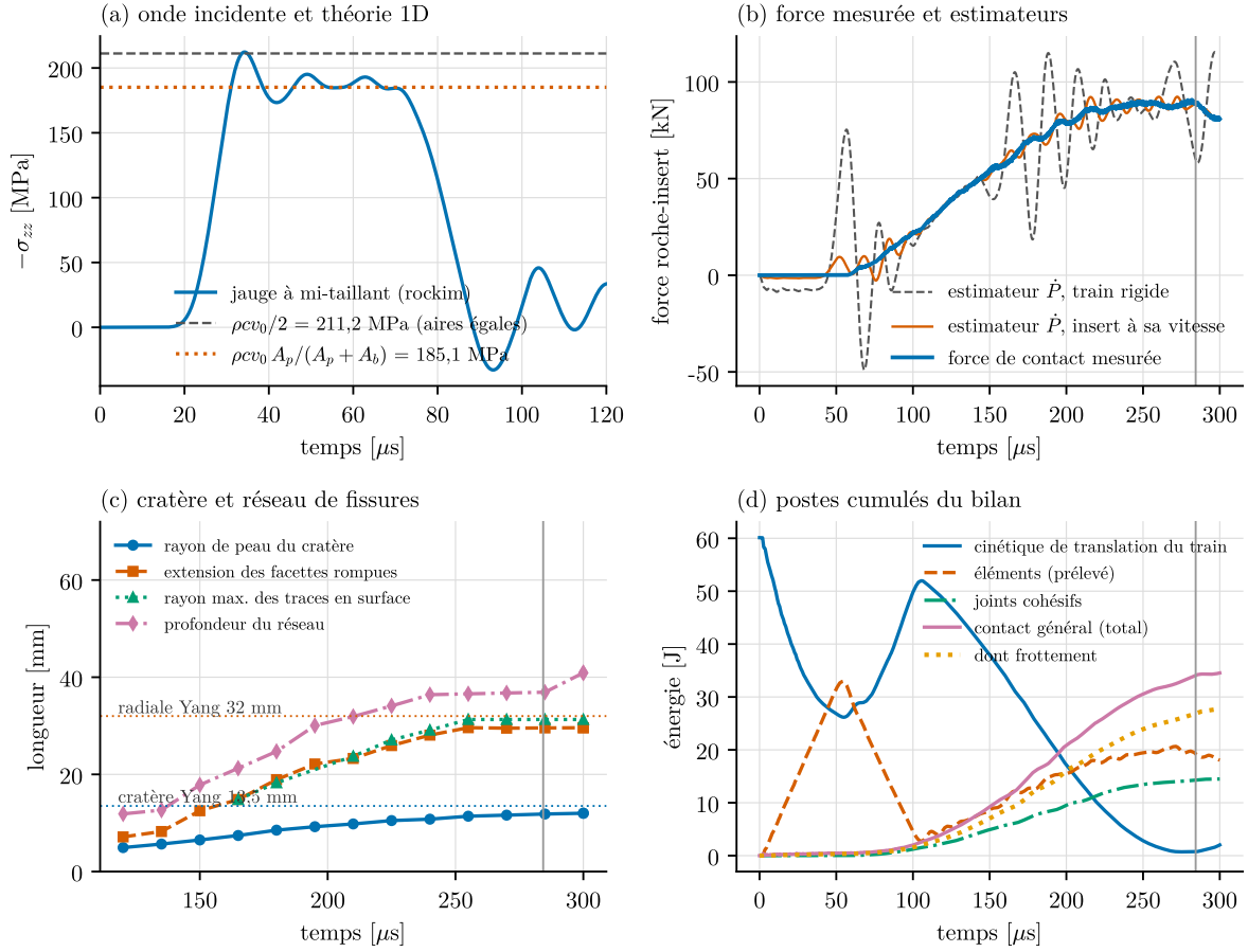
FIGURE 49 – Réplique St Anne : (a) onde à la jauge et théorie unidimensionnelle; (b) force insert-roche mesurée et estimateurs; (c) croissance du cratère et du réseau; (d) postes du bilan d'énergie. Trait vertical : fin de charge.
