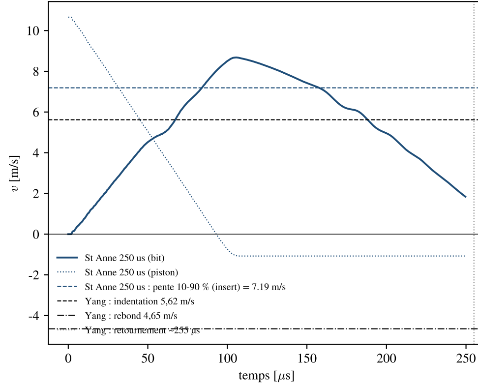
(b) Vitesse du bit et du piston, vers le bas > 0
