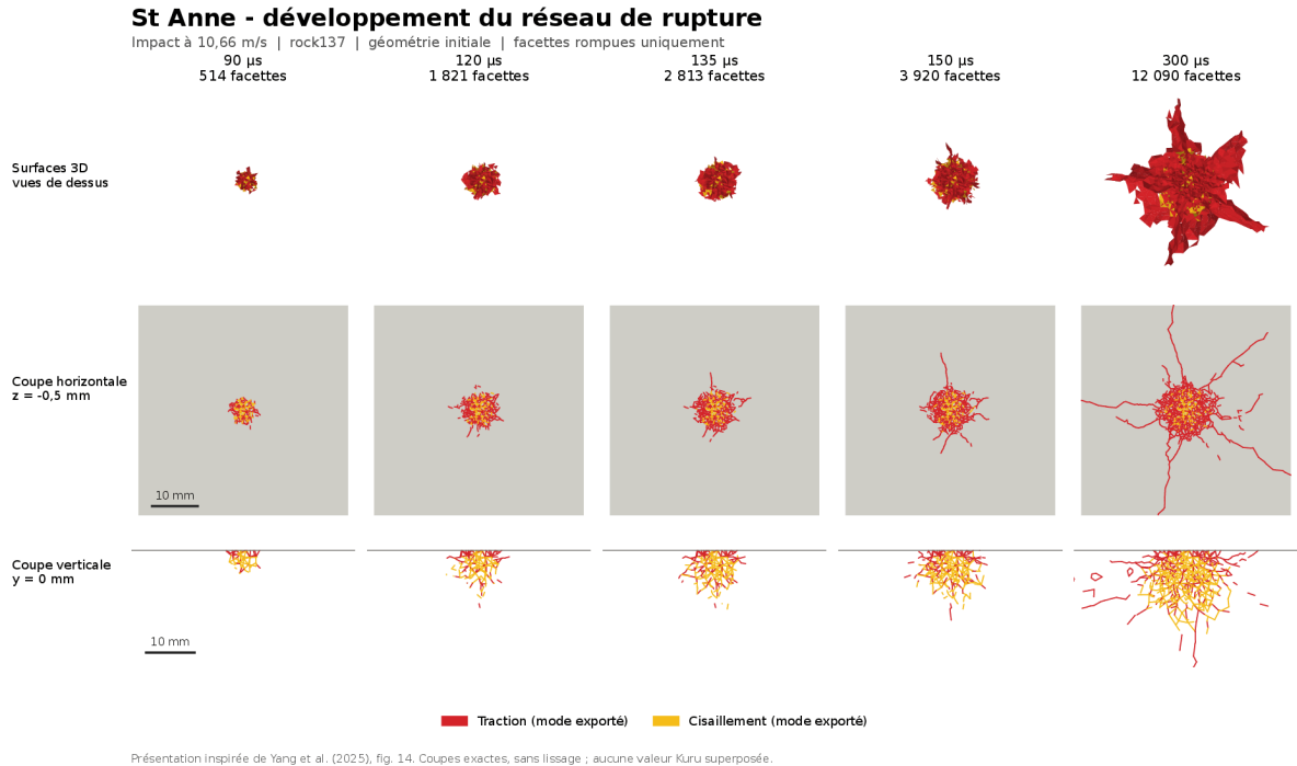
FIGURE 50 – Réplique St Anne : développement du réseau de facettes rompues de 90 à 300 \mu s, vu de dessus, en coupe horizontale à -0,5 mm et en coupe verticale ; couleur selon le mode de rupture.
