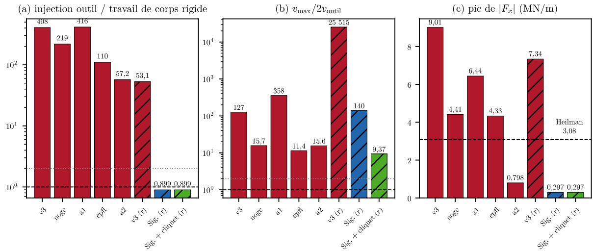
FIGURE 47 – Synthèse des runs de coupe d’août et du rejeu (r) : (a) rapport d’injection ; (b) vitesse nodale maximale rapportée à 2v , seuils 1 et 2 ; (c) pic de |F_x| contre la cible de Heilman.
