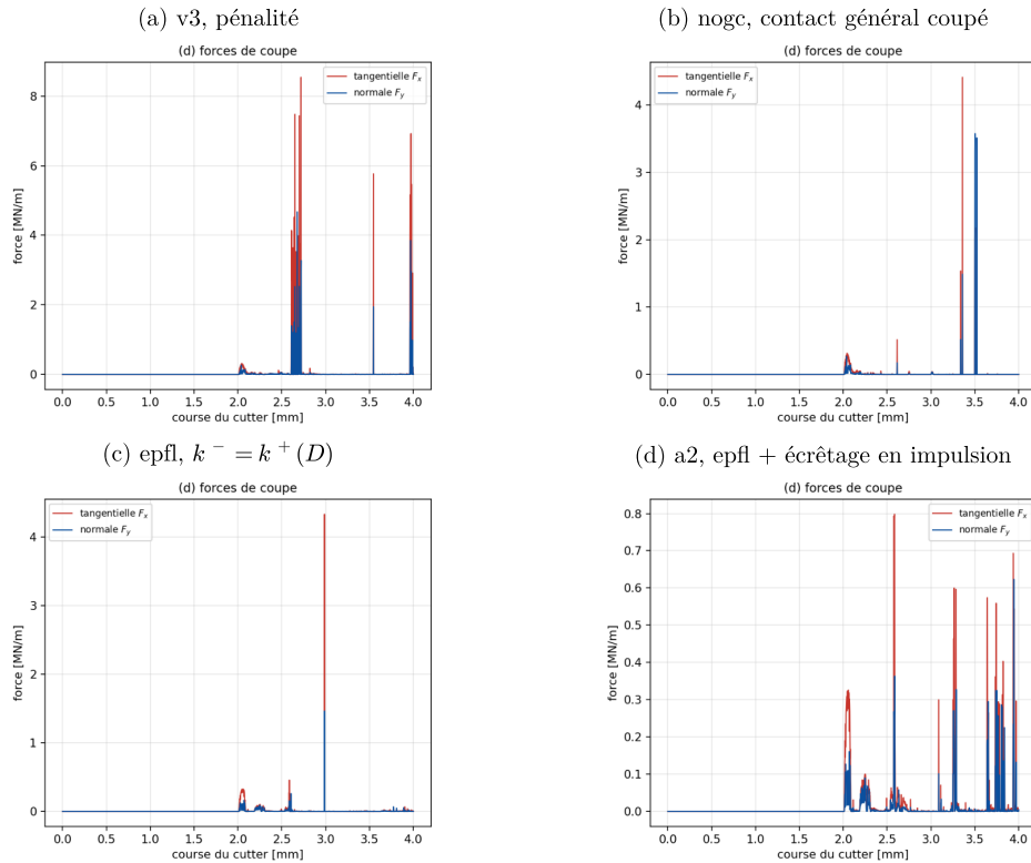
FIGURE 45 – Forces de coupe tangentielle (rouge) et normale (bleu) selon la course, runs d’août 2026, panneaux recadrés des planches d’archive : (a) v3 ; (b) contact général coupé ; (c) pénalité de compression EPFL ; (d) EPFL et écrêtage en impulsion.
