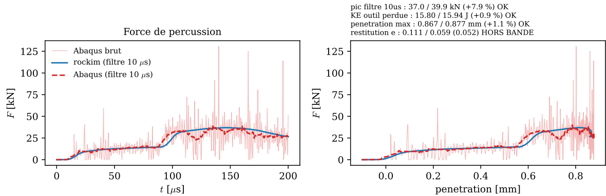
FIGURE 61 – Comparaison de code à code entre rockim et Abaqus/Explicit, loi de Saksala 2011, même maillage : force de percussion filtrée en fonction du temps et de la pénétration.
