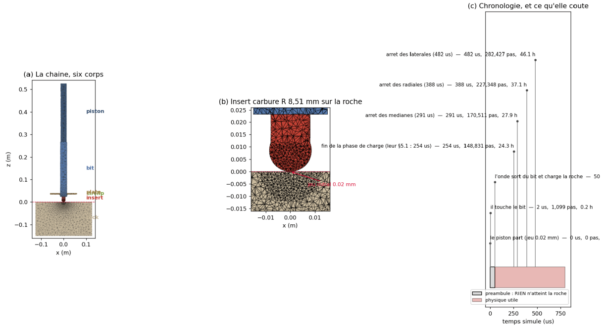
FIGURE 48 – Montage de la réplique St Anne : chaîne de six corps, insert en carbure posé à 0,02 mm de la roche, et coût en temps de calcul des événements de la chronologie.
