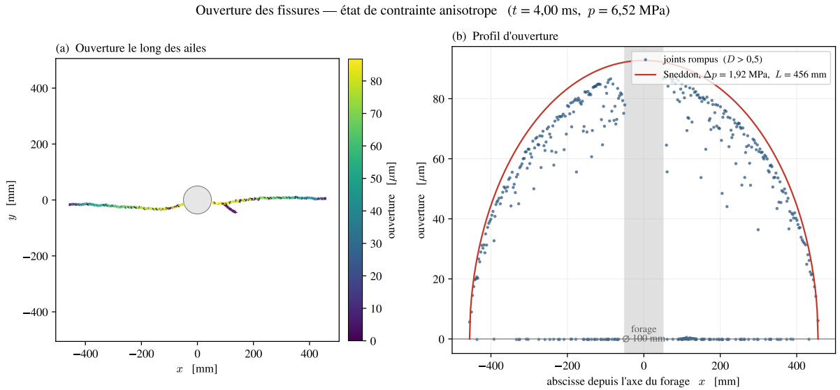
FIGURE 28 – Ouverture des fissures à t = 4 ms, état anisotrope, reconstruite lèvre à lèvre, et ellipse de Sneddon ( \Delta p = 1,92 MPa, L = 456 mm) : 89,0 \mu\text{m} mesurés pour 92,8 \mu\text{m} prédits. Les points à ouverture nulle sont des joints refermés.
