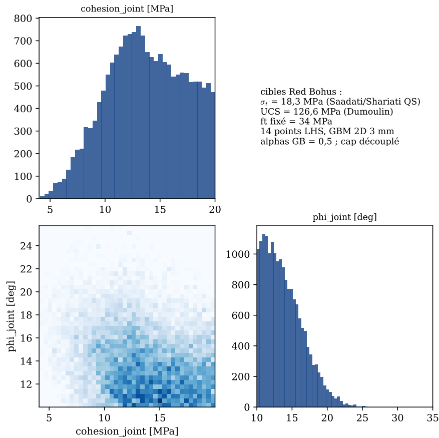
FIGURE 62 – Loi a posteriori de la calibration de juillet, modèle à grains 2D : angle de frottement des joints médian 13,4°, tronqué par la borne a priori ; cohésion peu contrainte.
