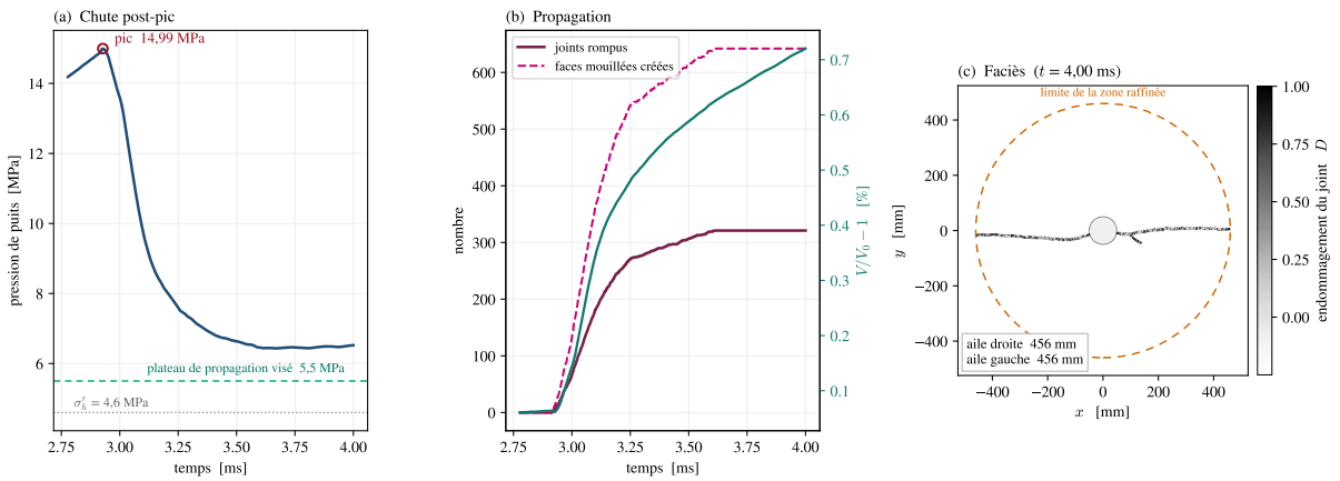
Phase post-pic — état de contrainte anisotrope ( \sigma'_H = 6,8 MPa, \sigma'_h = 4,6 MPa)
